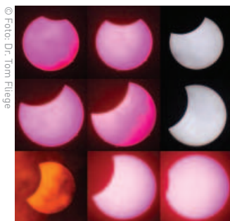
Partielle Sonnenfinsternis
