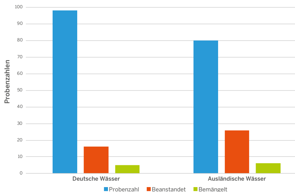
Abbildung 78: Anzahl der untersuchten Proben deutscher und ausländischer Wasser sowie beanstandete und bemängelte Probenzahlen
