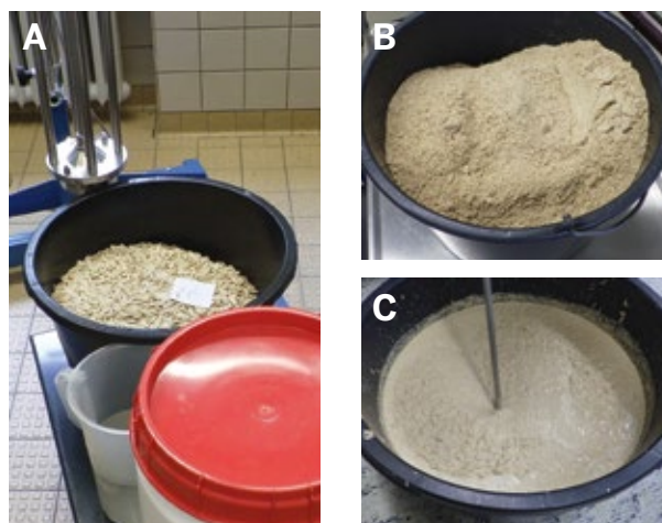
Abbildung 80: A – Größere Probenmenge Sonnenblumenkerne mit zur Nasshomogenisierung verwendetem Wasser sowie Chargenmischer. B – Vorgemahlene Probe Sonnenblumenkerne. C – Durchmischen eines „Slurrys“ aus vorgemahlene Sonnenblumenkernen nach Wasserzugabe
