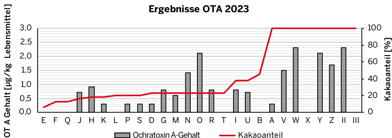
Abbildung 9: Graphische Übersicht über alle 2023 untersuchten kakaohaltigen Getränkepulver (A – U) sowie schwach (V – Z und II) und stark entölten Kakaopulver (III). Gehalte unterhalb der Nachweisgrenze (NG, 0,30 µg/kg) wurden als „null“ gewertet; Gehalte unterhalb der Bestimmungsgrenze (BG, 0,60 µg/kg), aber oberhalb der NG wurden mit der halben BG (entspricht 0,30 µg/kg) in die Darstellung mit aufgenommen
