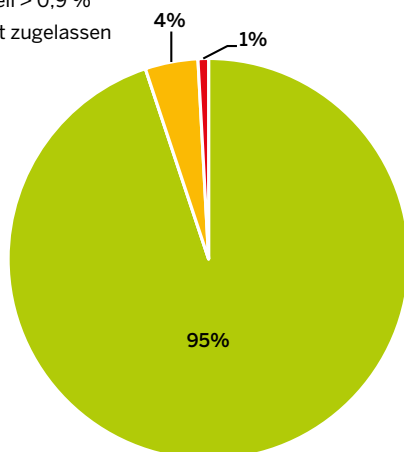
Abbildung 86: Ergebnisse der Untersuchung von Lebensmitteln auf gentechnisch veränderte Pflanzen in NRW im Jahr 2023
