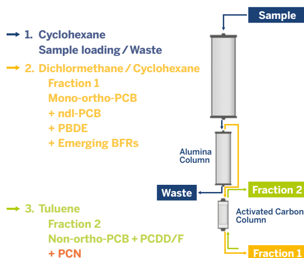
Abbildung 87: Aufarbeitungsschema der Multimethode hPOPs
