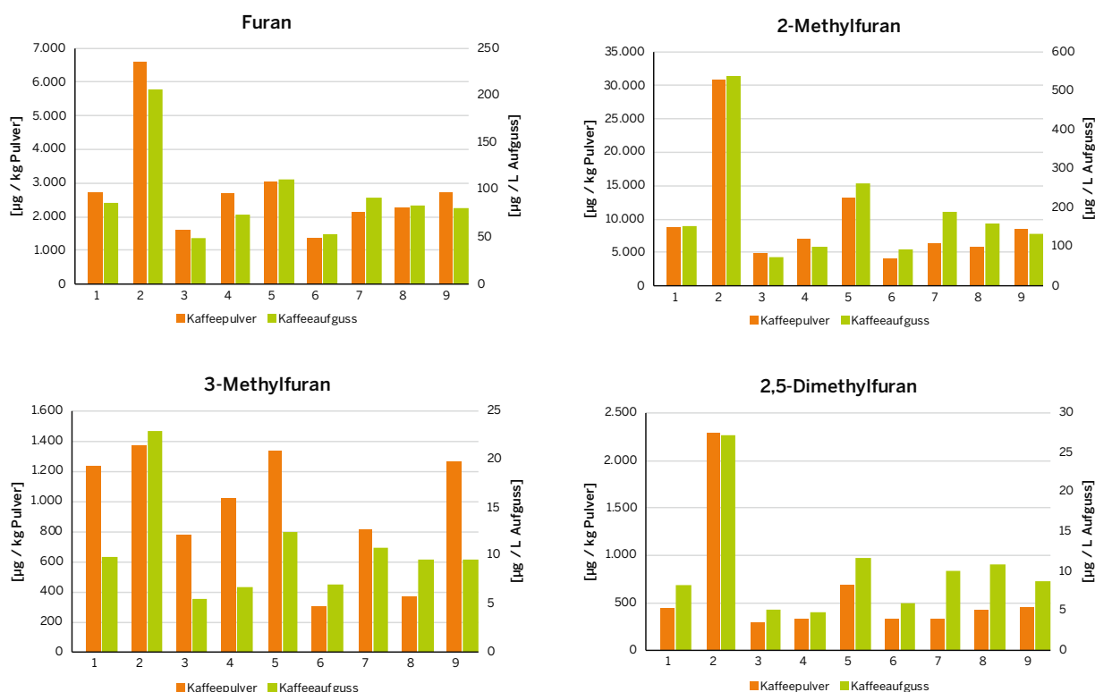
Abbildung 77: Ergebnisüberblick der nachgewiesenen Gehalte (Mittelwerte aus Doppelbestimmung) an Alkylfuranen und Furan in ausgewählten Kaffeepulvern (Gehalt in \mu\text{g/kg} Pulver) und daraus aufgebrühten Kaffeeaufgüssen (Gehalt in \mu\text{g/L} Aufguss) ( n = 9 )
