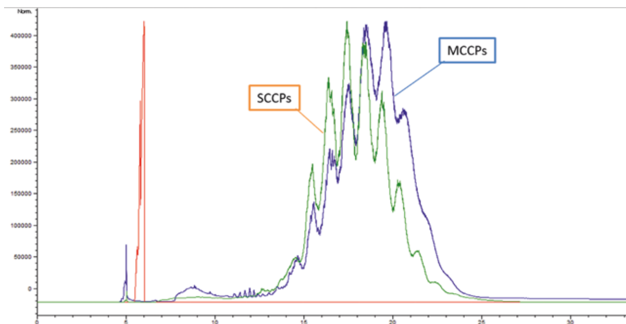
Abbildung 88: TIC-Chromatogramm eines CP-Standards: SCCP (short-chained chlorinated paraffins) und MCCP (Medium-chained chlorinated paraffins)
