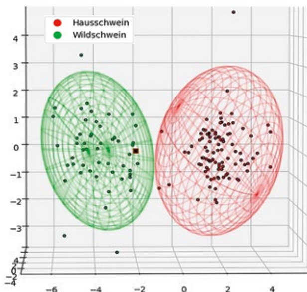
Abbildung 35: Scoreplot der linearen Diskriminanzanalyse für Fleischproben mit der Angabe „Wildschwein“ bzw. „Hausschwein“ und eine zu prüfende Routineprobe „Wildschweingulasch“ (quadratisch dargestellt)
