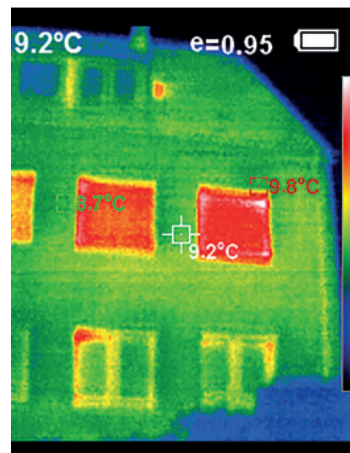
Wärmebild der Fenster vor dem Austausch: Erdgeschoss neu und Obergeschoss alt
