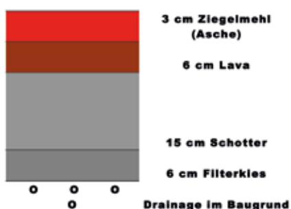
Aufbau eines Ziegelmehlplatzes nach DIN 18035 Teil 5:
