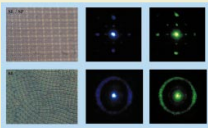
Abb. 8: Durch Polymerisation fixierte Muster eines chiral-nematischen Flüssigkristalls (links) und das jeweilige Beugungsbild (rechts). Oben: Probe mit einheitlicher Randerorientierung. Unten: Probe ohne spezielle Randerorientierung.
