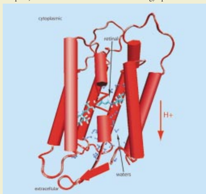
Abb. 4: Bacteriorhodopsin mit eingebettetem optisch aktivem Retinal-Molekül, A-G: \alpha -Helixen.
