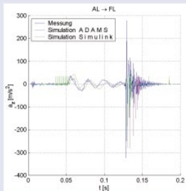
Abb. 6: Simulation und Messung beim Schalten des Bi-Xenon-Reflexionssystems.
