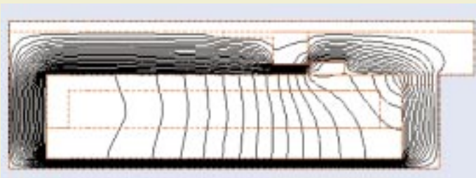
Abb. 4: Feldlinienverteilung des Hubmagneten mit kennlinienoptimierter Luftspaltgeometrie.
