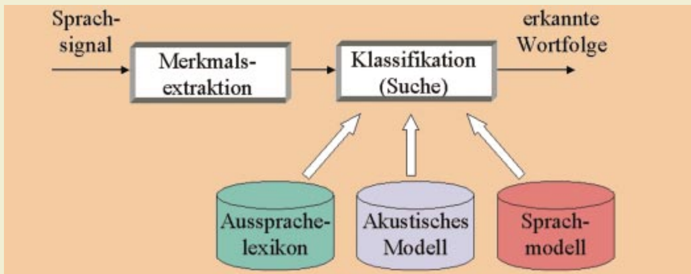
Abb. 1: Blockschaftbild eines Spracherkenners.
