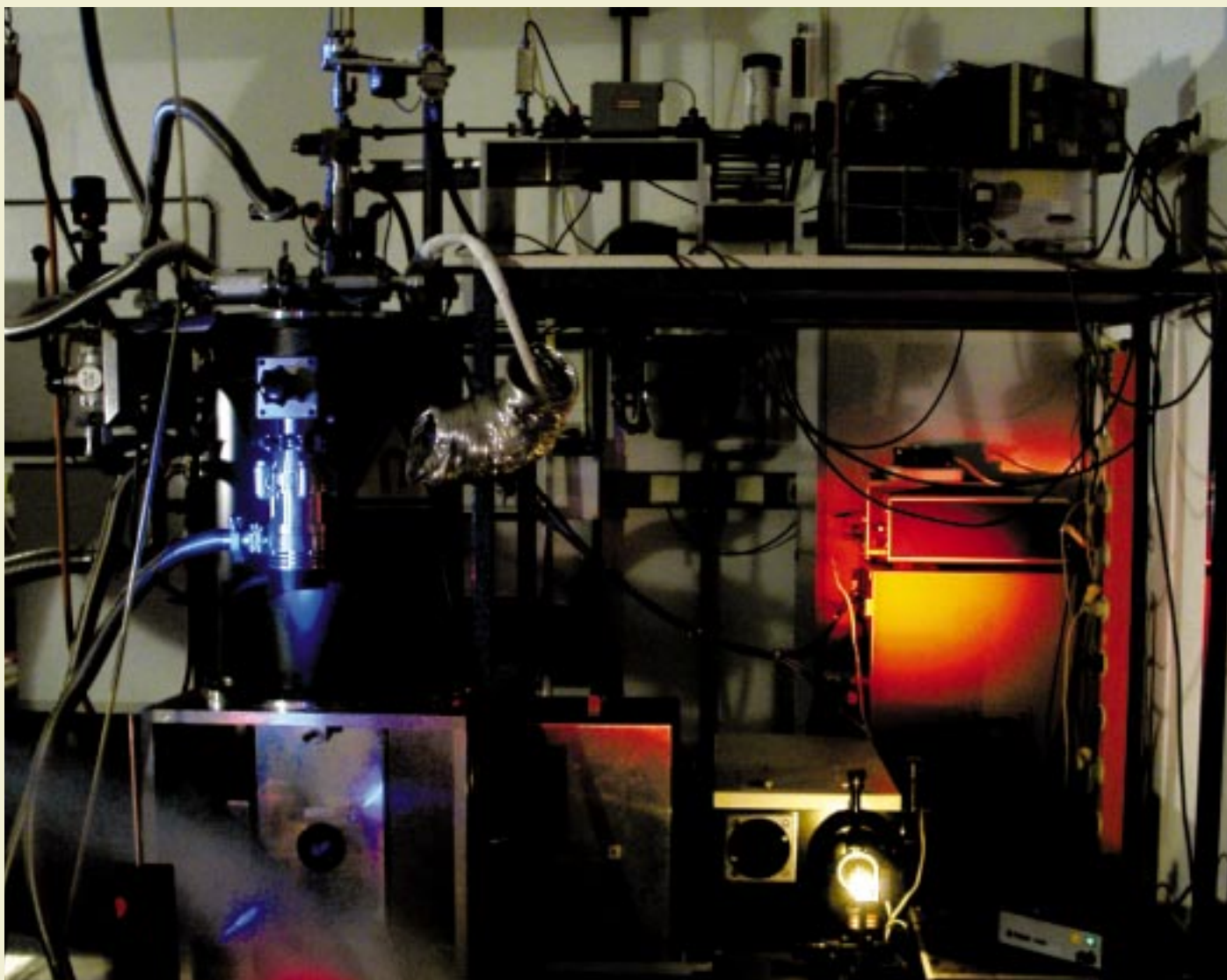
Abb. 3: Apparatur zum optischen Nachweis der elektronenparamagnetischen Resonanz. In dem blau beleuchteten Kryostaten befindet sich ein heliumgekühlter supra-leitender Magnet zur Erzeugung des statischen Magnetfeldes bis 5 Tesla.
