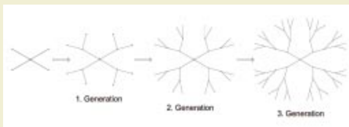
Abb. 1: Dendrimmerwachstum der ersten, zweiten und dritten Generation.
