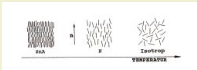
Abb. 3: Anordnung stäbchenförmiger Moleküle in verschiedenen Phasen. „SmA“: flüssigkristalline, smektische A-Phase, „N“: flüssigkristalline, nematische Phase, „iso“: normale, isotrope Flüssigkeit.
