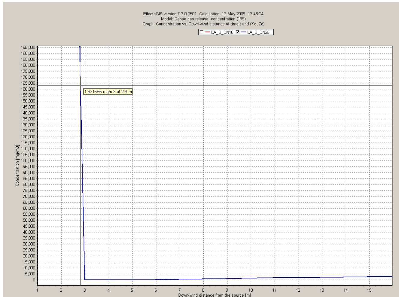
Diagramm A4.3-7: CO 2 -Konzentrationsprofil in Atemhöhe 1,5 m bei Stützenabriss DN25 (Markierung = 9 Vol.-% CO 2 )
