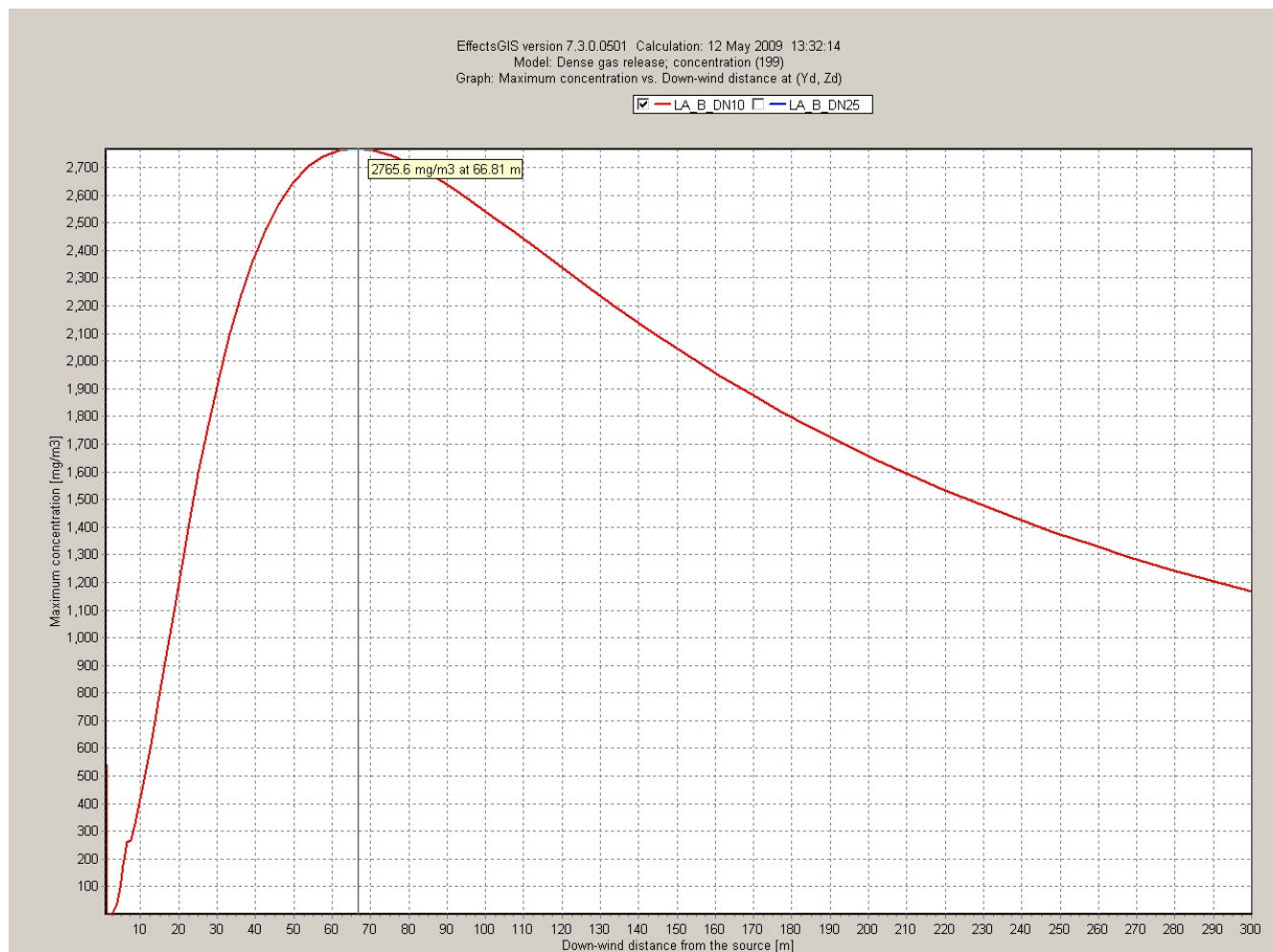
Diagramm A4.3-1: CO 2 -Konzentrationsprofil in Atemhöhe 1,5 m bei Stutzenabriss DN10 (Markierung = max. Konzentration)
