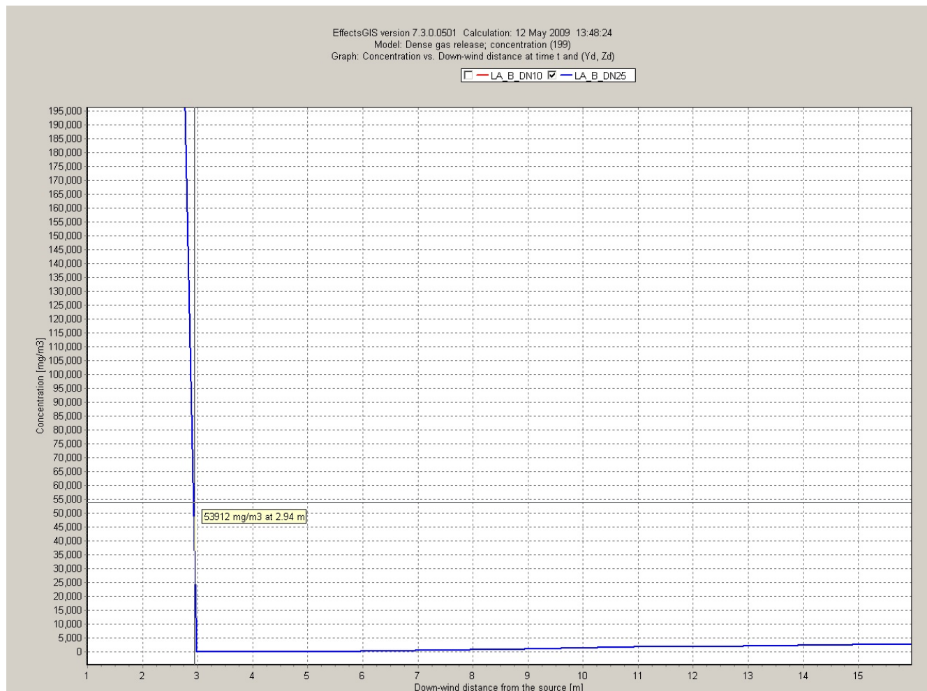
Diagramm A4.3-8: CO 2 -Konzentrationsprofil in Atemhöhe 1,5 m bei Stützenabriss DN25 (Markierung = TEEL-2-Wert)
