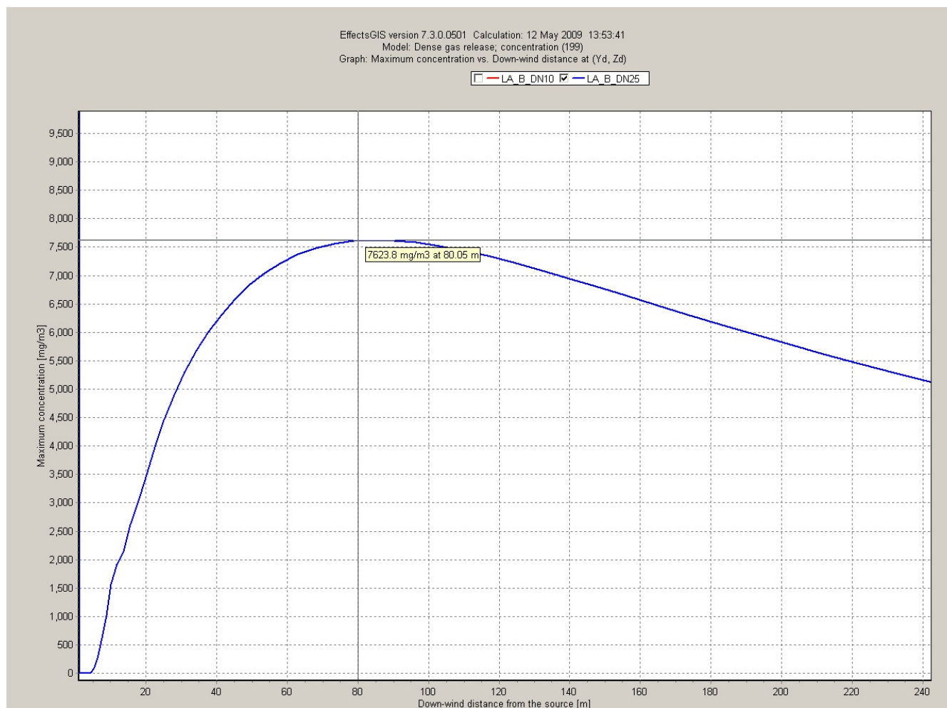
Diagramm A4.3-2: CO 2 -Konzentrationsprofil in Atemhöhe 1,5 m bei Stützenabriss DN25 (Markierung = max. Konzentration)
