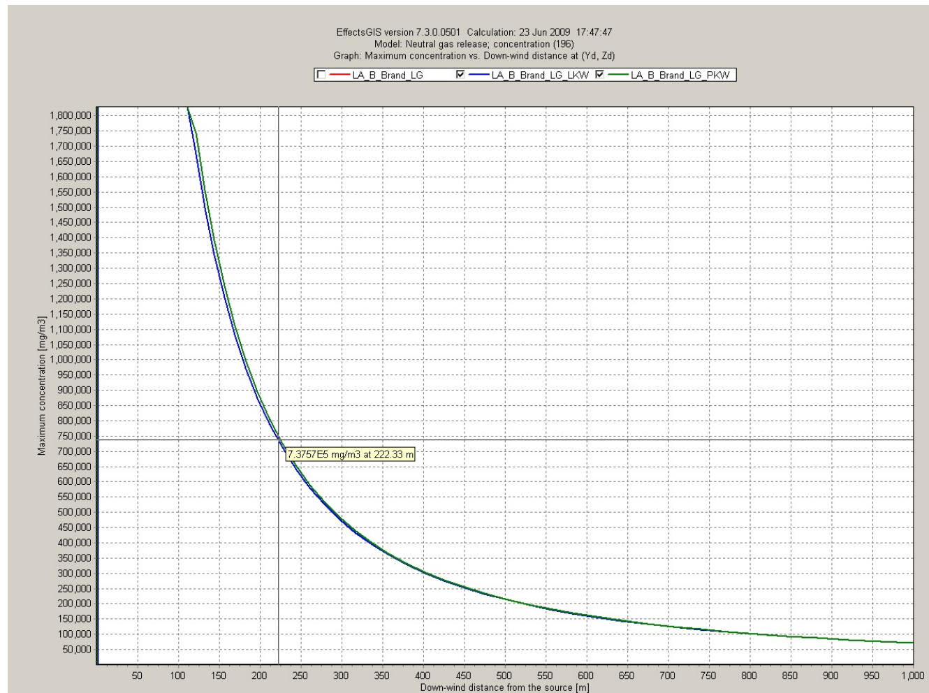
Diagramm A4.3-13: CO 2 -Konzentrationsprofil für Fahruntüchtigkeit von LKW (0,8 m über Erdgleiche) bei ordnungsgemäßer Auslösung
