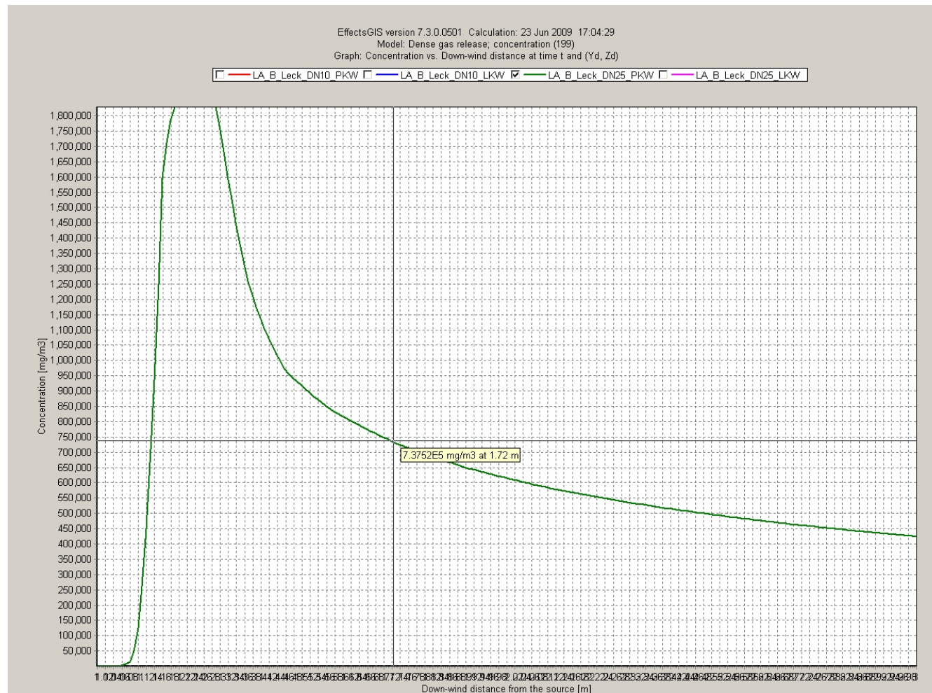
Diagramm A4.3-6: CO 2 -Konzentrationsprofil für Fahruntüchtigkeit von PKW (0,2 m über Erdgleiche) bei Stutzenabriss DN25
