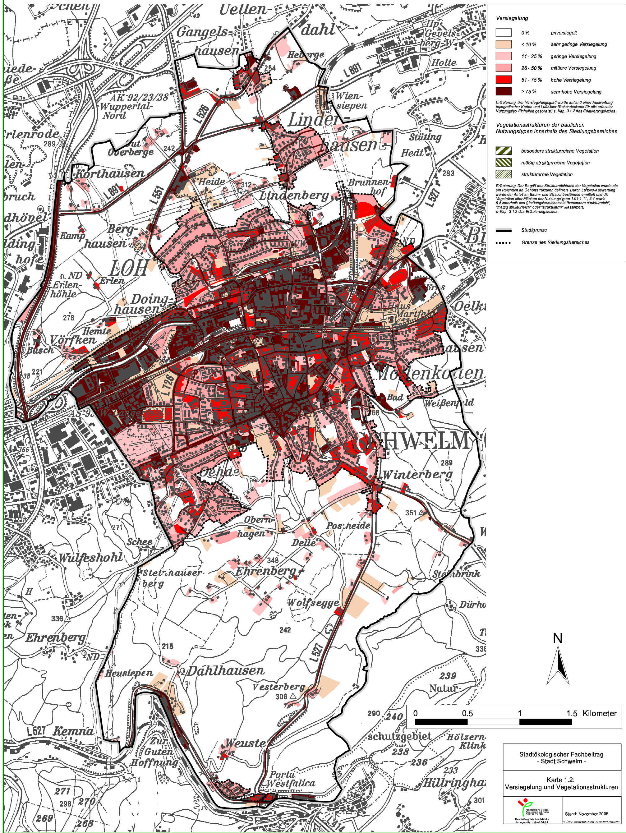
Karte 1.2: Versiegelung und Vegetationsstrukturen
