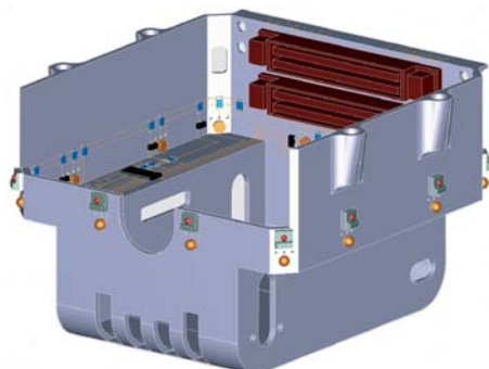
MID-Gehäuse eines Miniroboters
