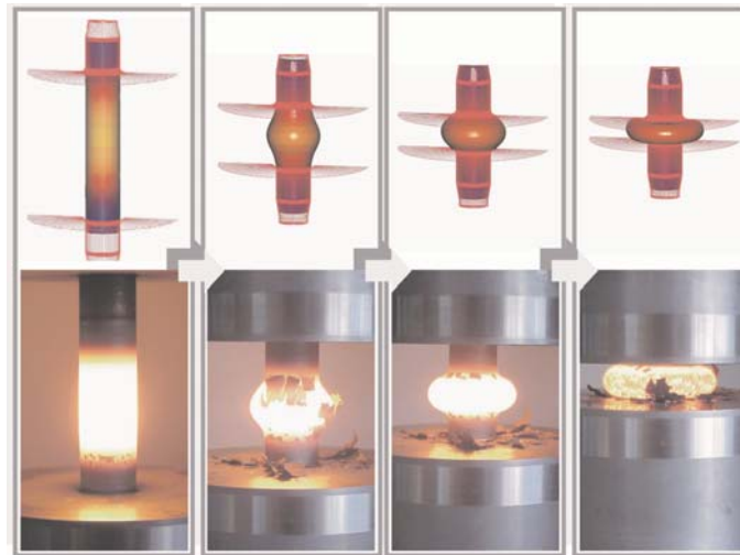
Virtueller und realer Prozessverlauf einer simultanen Kalt- und Warmumformung zur Herstellung einer Welle mit gradierten Eigenschaften
