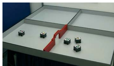
Überprüfung der entwickelten Regelstrategien im Experiment auf der Telewerkbank
