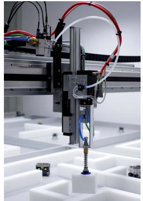
Der Greifarm kann Roboter und Bausteine greifen und so verschiedene Szenarien in kürzester Zeit reproduzierbar aufbauen.
