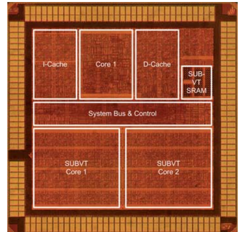
Chipfoto des Prozessors CoreVA ULP
