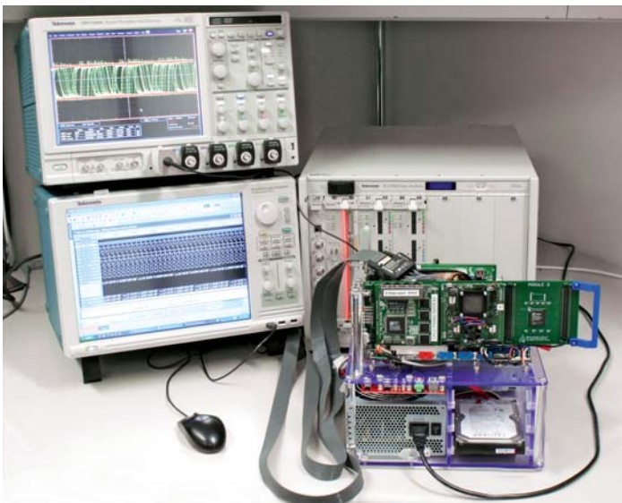
Testaufbau für die Charakterisierung des im Heinz Nixdorf Institut entwickelten Prozessorkerns CoreVA ULP
