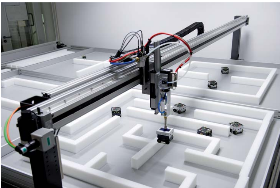
Die neue Telewerkbank im Robotiklabor des Heinz Nixdorf Instituts
