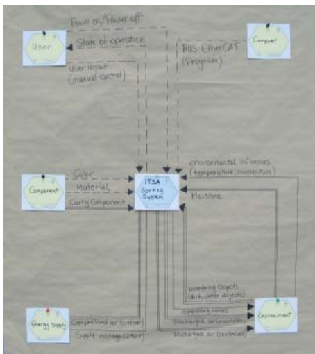
Umfeldmodell der Sortieranlage
