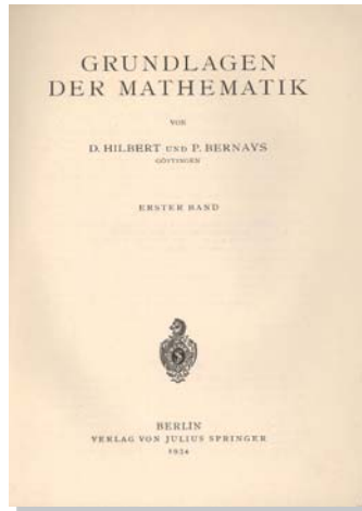
Titelblatt Hilbert/Bernays
