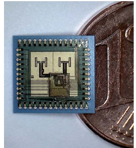
Der neue Radarsensor ist nur halb so groß wie eine Eurocent-Münze, aber beinhaltet ein komplettes Radarsystem mit Antennen. (Bild: Robert Bosch GmbH/SUCCESS)
