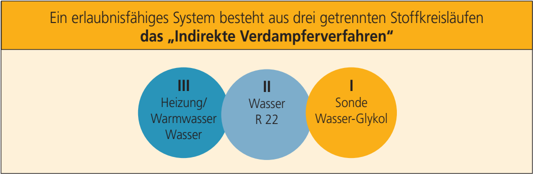
[Bild 19] System Erdwärmanlage
