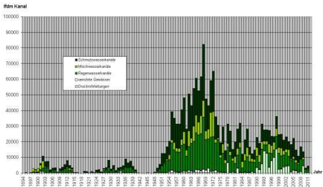
Abbildung 1: Baujahre des Kanalnetzes – Stand 31.12.2011
