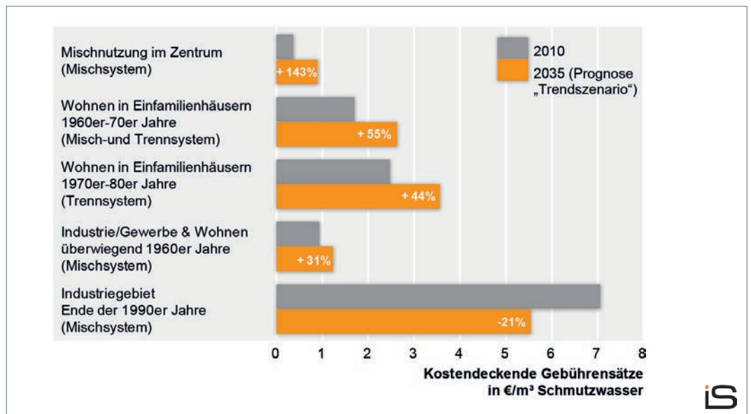
Quartiersspezifische Kosten der Abwasserkanalisation im Vergleich
