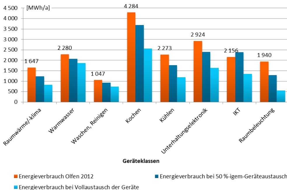
Abbildung 5-8: Potenzial zur Minderung des Strombedarfs der Haushalte in Olfen durch Gerätetausch
