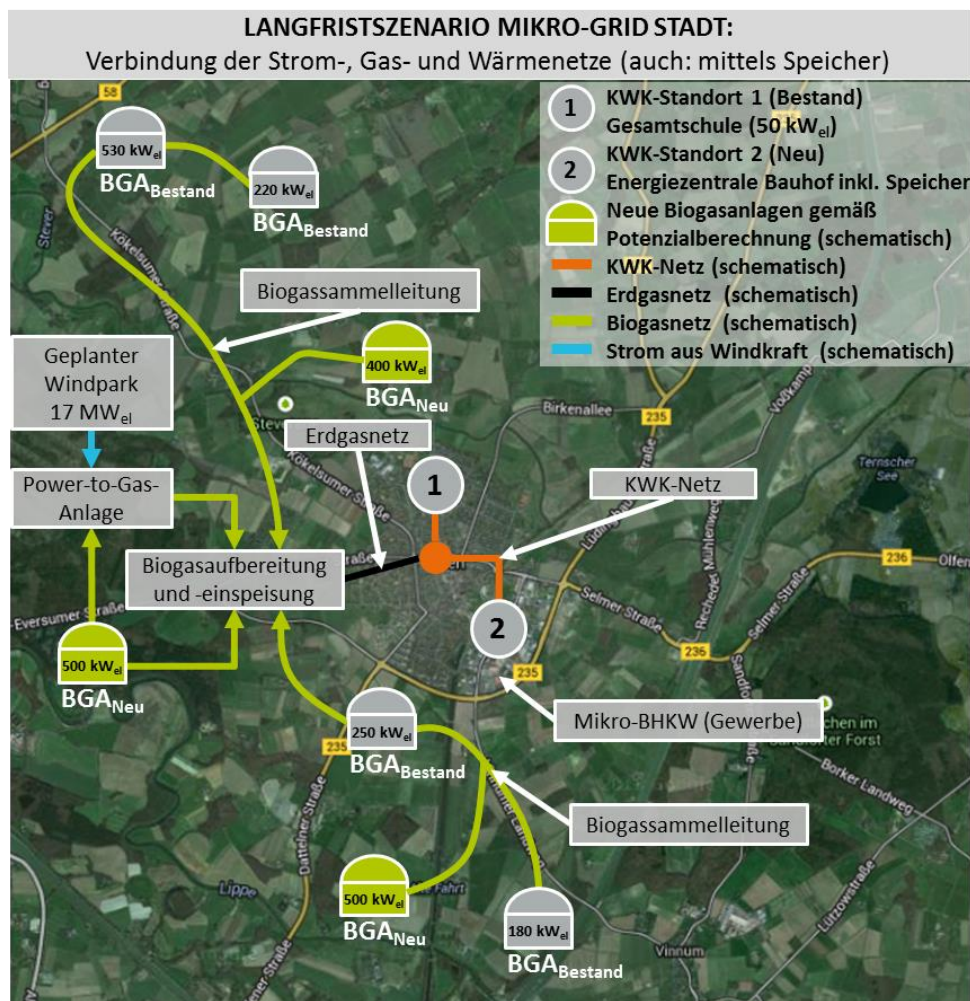
Abbildung 7-1: Technische Potenziale zur Umsetzung der Energievision Olfen
