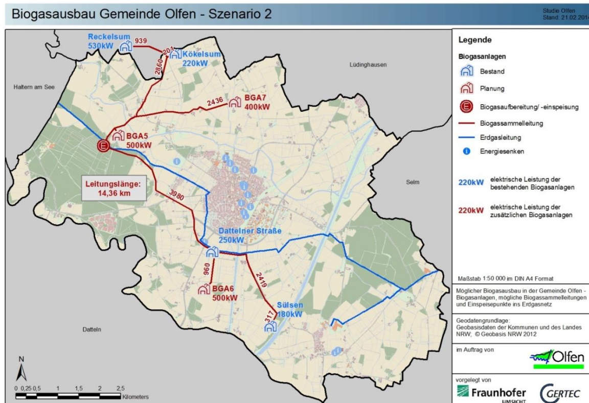
Abbildung 5-5: Biogassammelleitung des Szenario 2 im GIS-Modell
