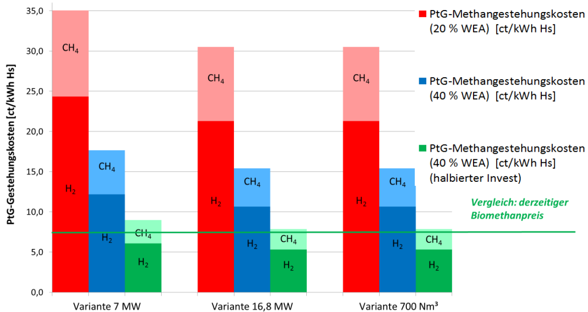
Abbildung 5-2: Gestehungskosten der Power-to-Gas-Nutzung
