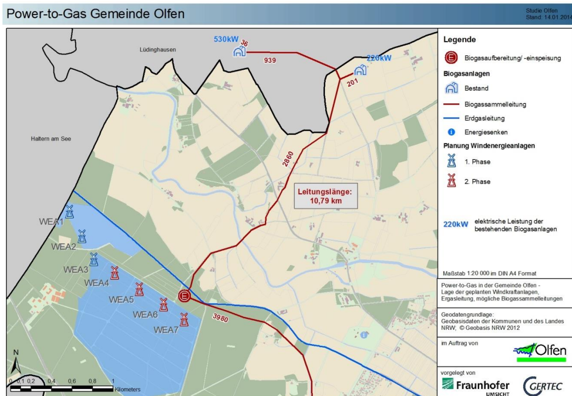
Abbildung 5-1: Mögliche Windkraft- und Power-to-Gasstandorte im GIS-Modell
