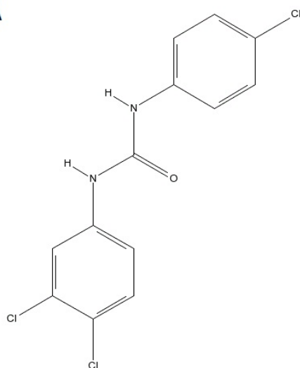
Abbildung 3: Darstellung von zwei angebotenen SMILES für Triclocarban als Molekülzeichnung (Tabelle 5); A: korrekter SMILES aus Chemicalize; B: fehlerhafter SMILES aus der Chemspider Datenbank, bei dem die Position eines Wasserstoffatoms verschoben ist
