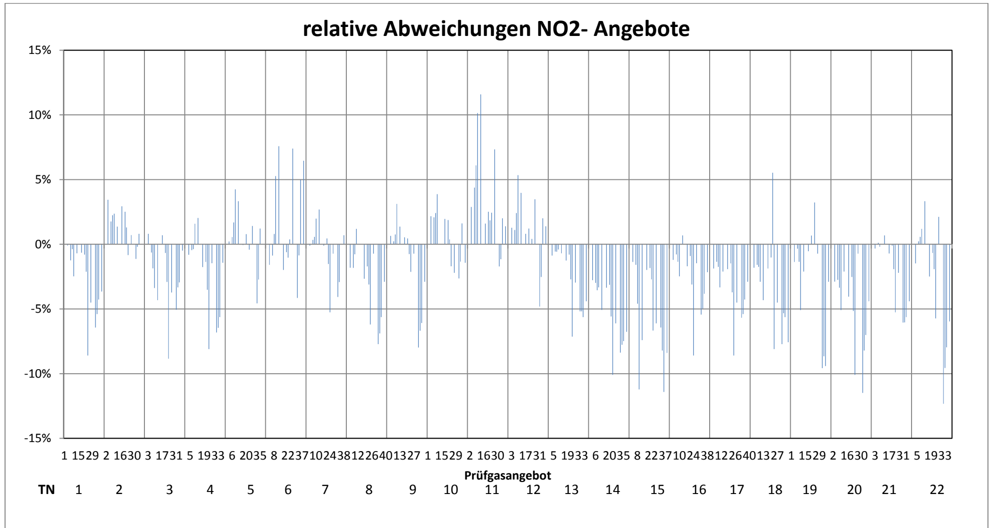
Abbildung 20: Relative Abweichungen der Teilnehmermesswerte des Ergänzungsteiles für die Komponente NO2
