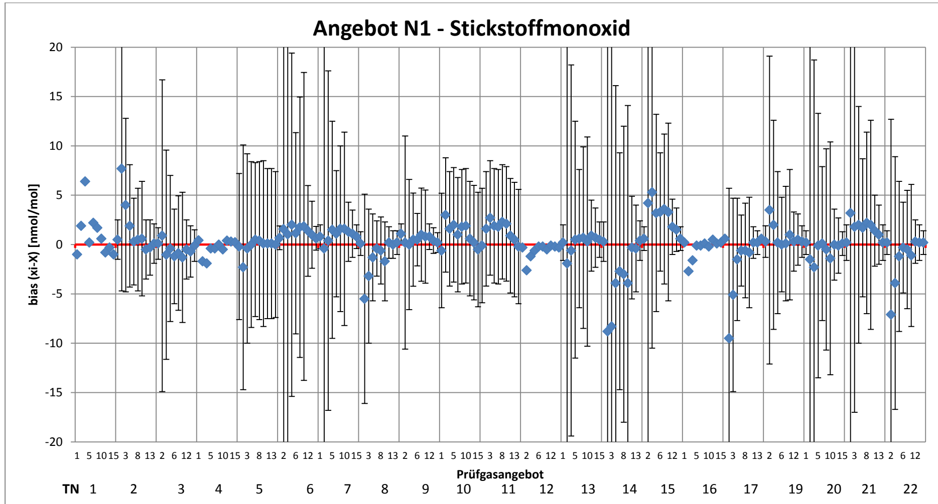
Abbildung 17: Abweichungen und erweiterte Unsicherheiten der Teilnehmermesswerte - Angebote N1 für die Komponente NO
