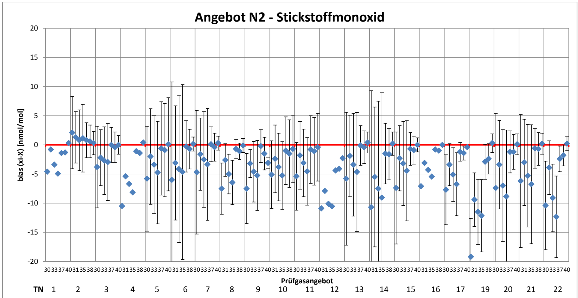
Abweichungen und erweiterte Unsicherheiten der Teilnehmermesswerte - Angebote N2 für die Komponente NO
