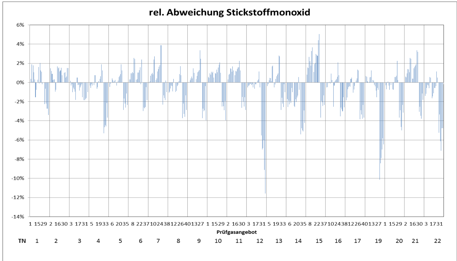
Abbildung 16: Relative Abweichungen der Teilnehmersmesswerte des Ergänzungsteiles für die Komponente NO
