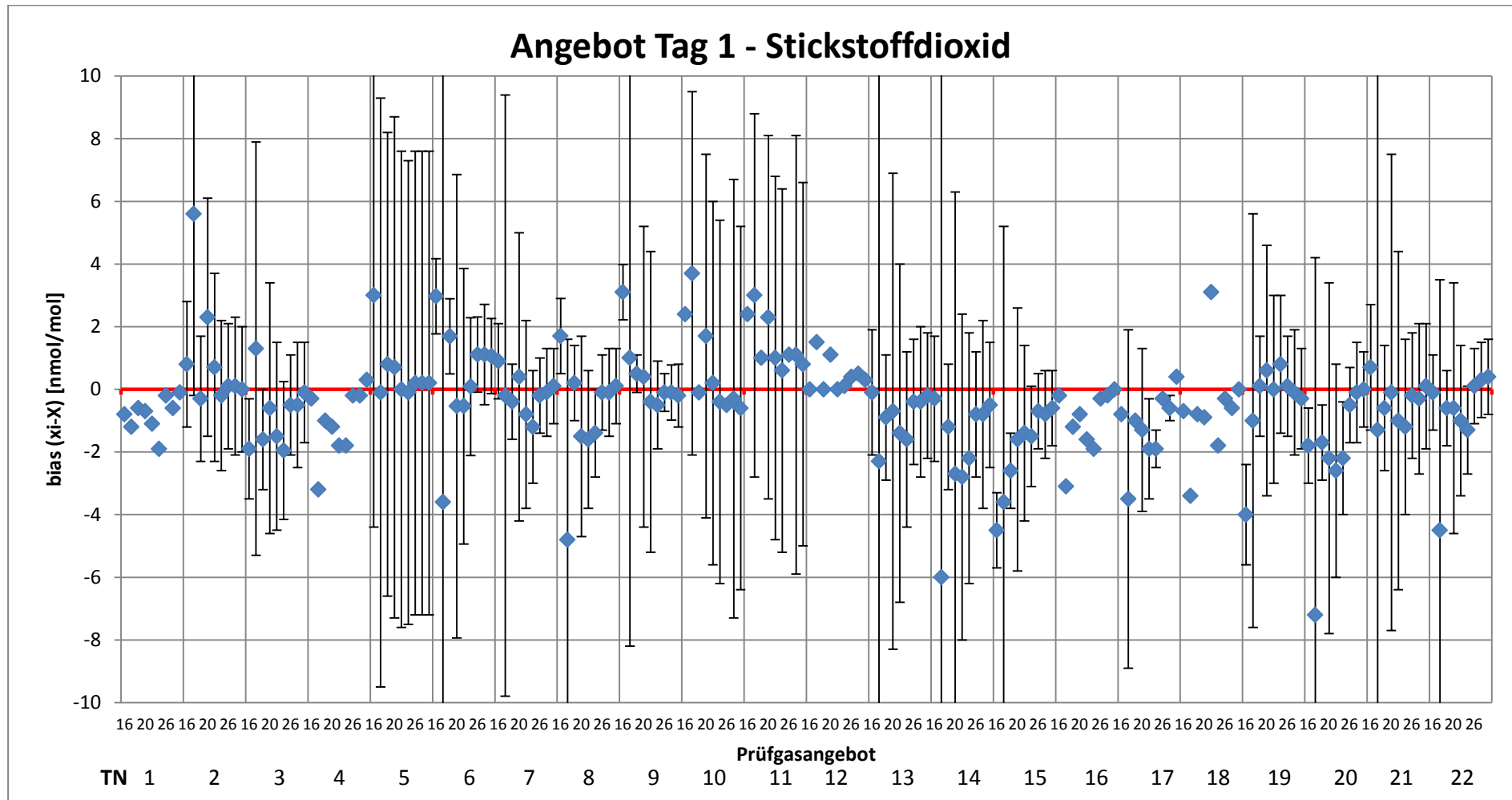
Abbildung 22: Abweichungen und erweiterte Unsicherheiten der Teilnehmersmesswerte - Angebote Tag 1 für die Komponente NO 2
