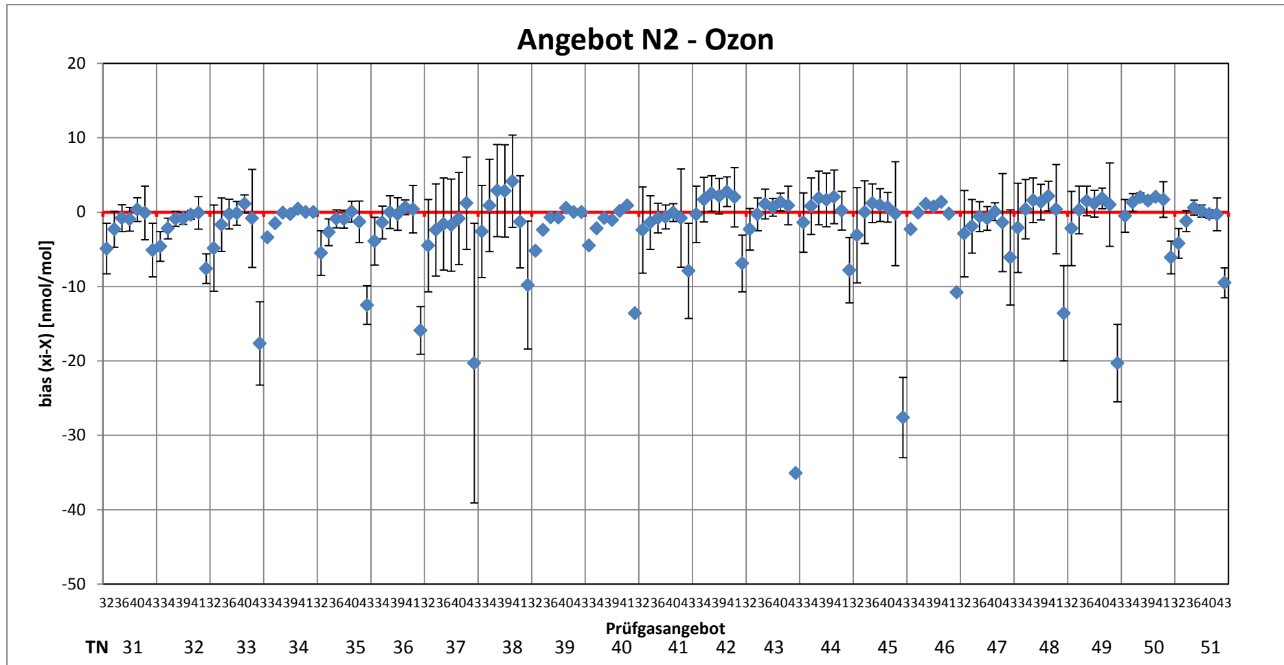
Abbildung 27: Abweichungen und erweiterte Unsicherheiten der Teilnehmersmesswerte - Angebote N2 für die Komponente Ozon
