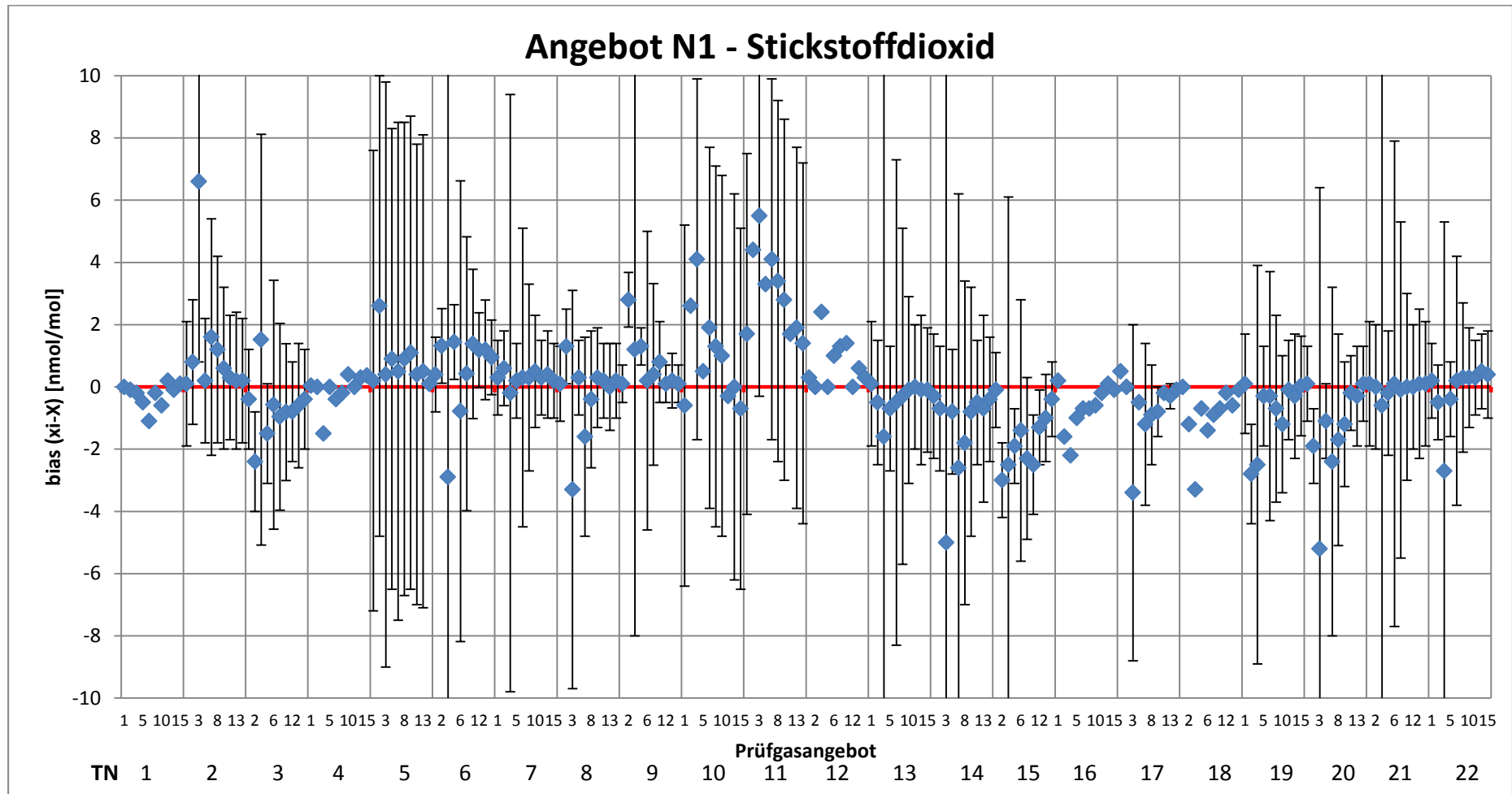
Abbildung 21: Abweichungen und erweiterte Unsicherheiten der Teilnehmermesswerte - Angebote N1 für die Komponente NO 2
