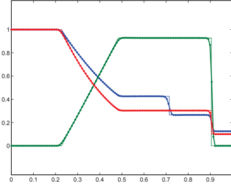
(d) HLL- P_1 -Q, E_2^p=9.56\text{e-}5
