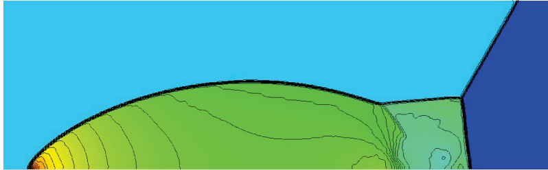
(d) HLL- P_1 -Q, p \in [1.0, 543.68]
