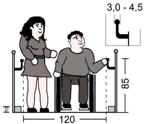
Rampe, Querschnitt
