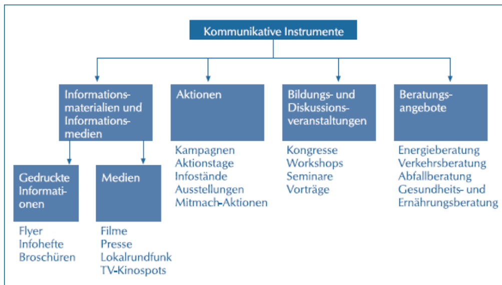
Abb. 24: Kommunikative Instrumente 31
