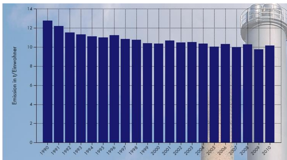
Abb. 12: Entwicklung pro-Kopf CO 2 -Ausstoß in Deutschland 1990-2010 10
