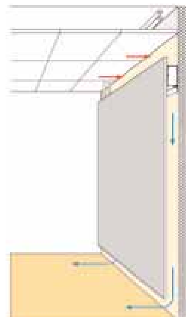
Abb. 8-2: Funktionsprinzip des Schwerekräftsystems für den Kühlfall
