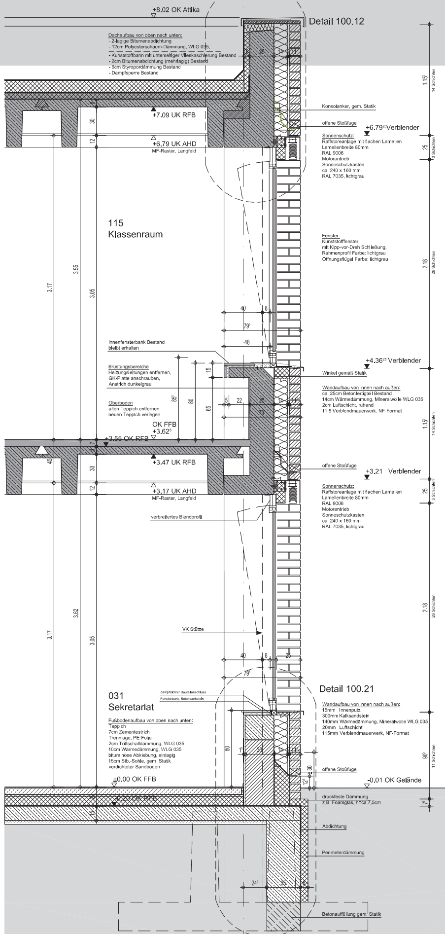
Fassadenschnitt 2-2
