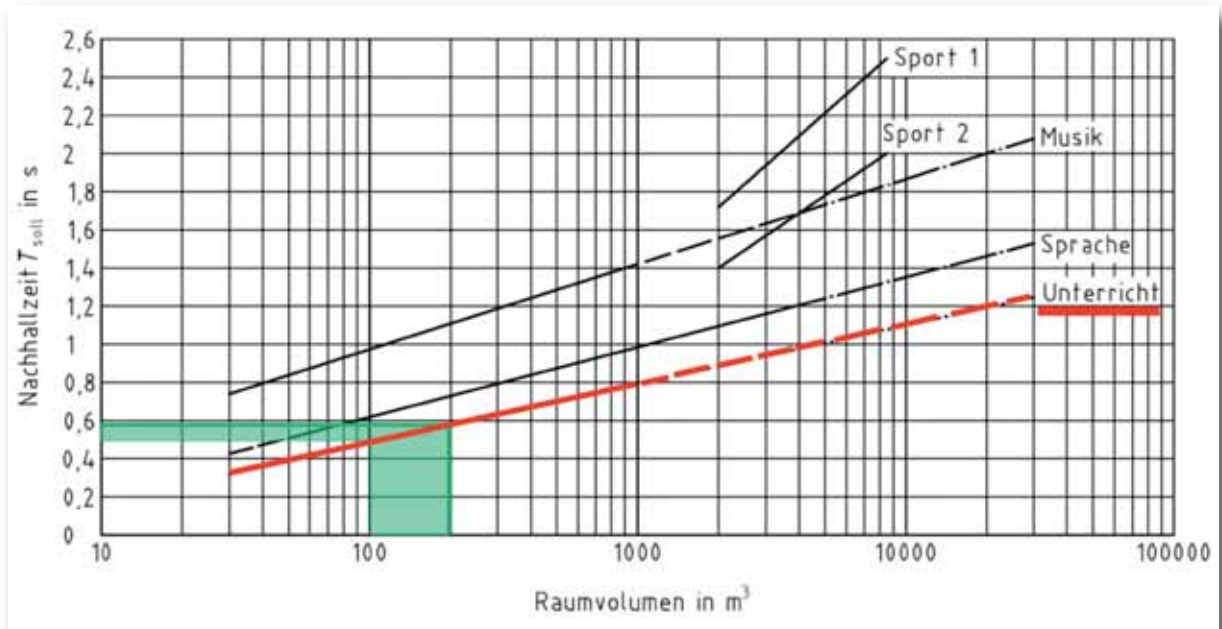
Abb. 9-1: Sollwert der Nachhallzeit für unterschiedliche Nutzungsarten 21
