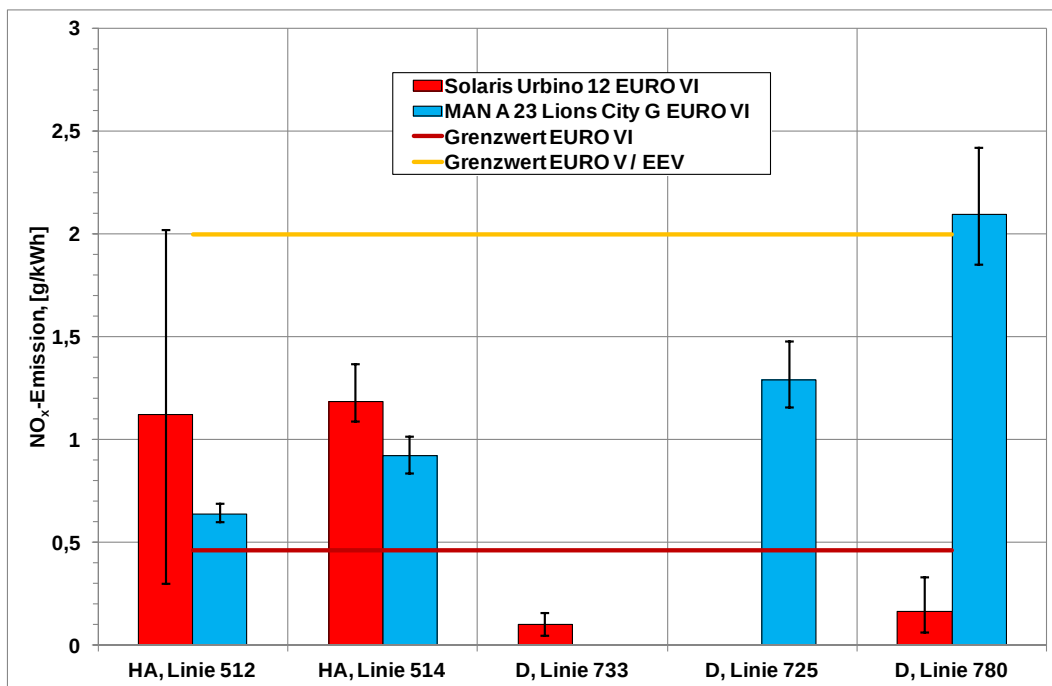
Abbildung 32: Übersicht der mittleren \text{NO}_x -Emissionen bei Betrieb im Realverkehr im Vergleich zum \text{NO}_x -Emissionsgrenzwert.
