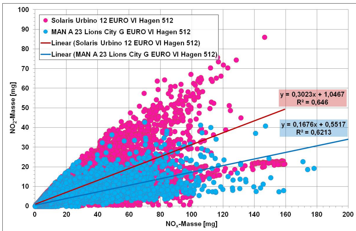
Abbildung 30: \text{NO}_x - und \text{NO}_2 -Massen auf der Linie 512, Hagen
