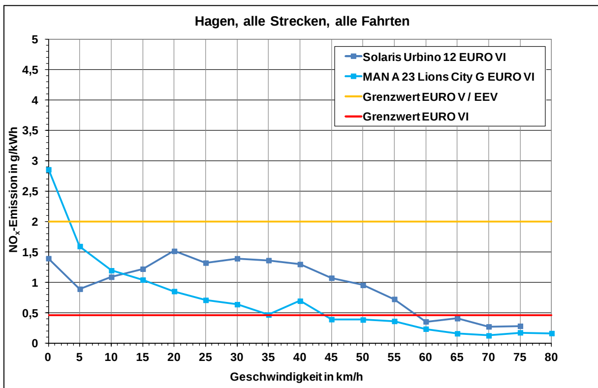
Abbildung 20: NO x -Emissionen in [g/kWh] in Abhängigkeit von der Geschwindigkeit, Einsatzgebiet Hagen
