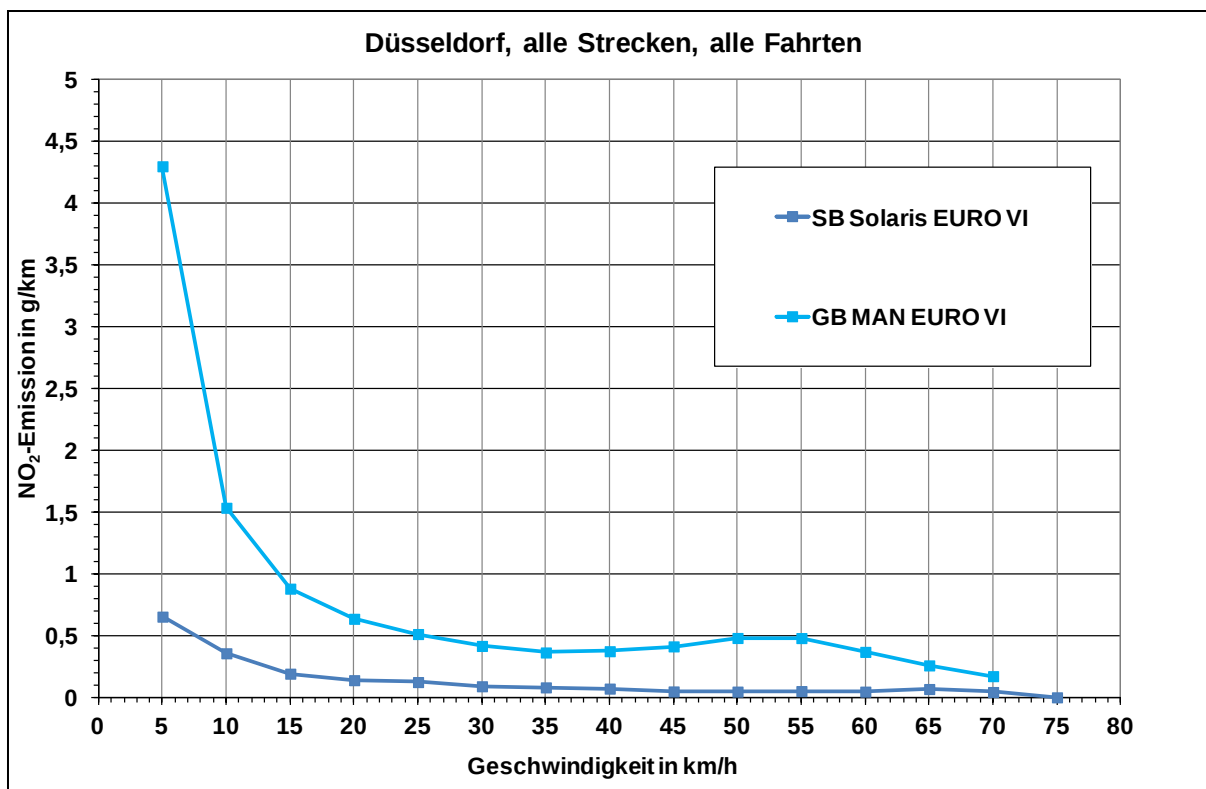
Abbildung 26: NO 2 -Emissionen in [g/km] in Abhängigkeit von der Geschwindigkeit, Einsatzgebiet Düsseldorf
