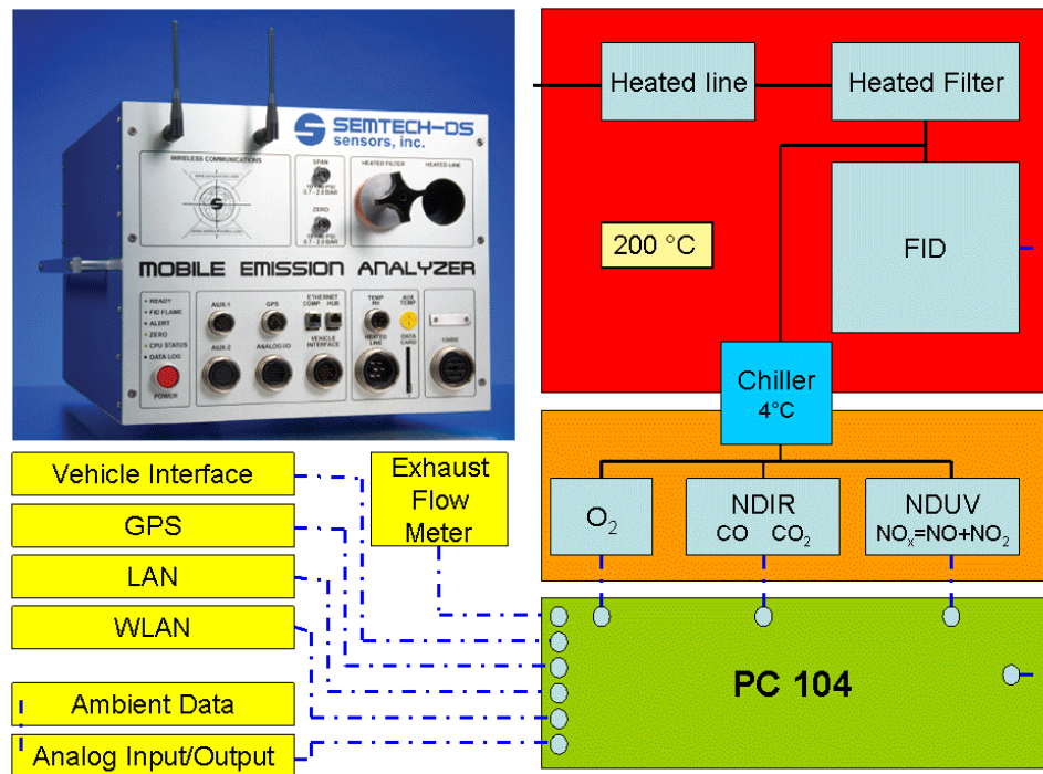
Abbildung 8: Semtech-DS-Messgerät [Quelle: Sensors]
