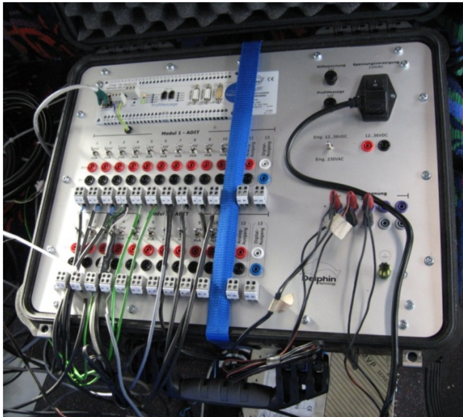
Abbildung 13: Datalogger für zusätzliche Messsignale
