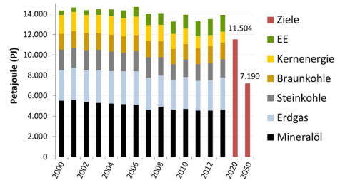
5// Entwicklung des Primärenergieverbrauchs in Deutschland nach Energieträgern mit Zielen. 12
