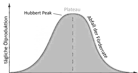
2// Schema einer Förderkurve nach dem Geologen Hubbert. Gestrichelte Linie = Punkt an dem 50% der Quellen gefördert wurden. 4
