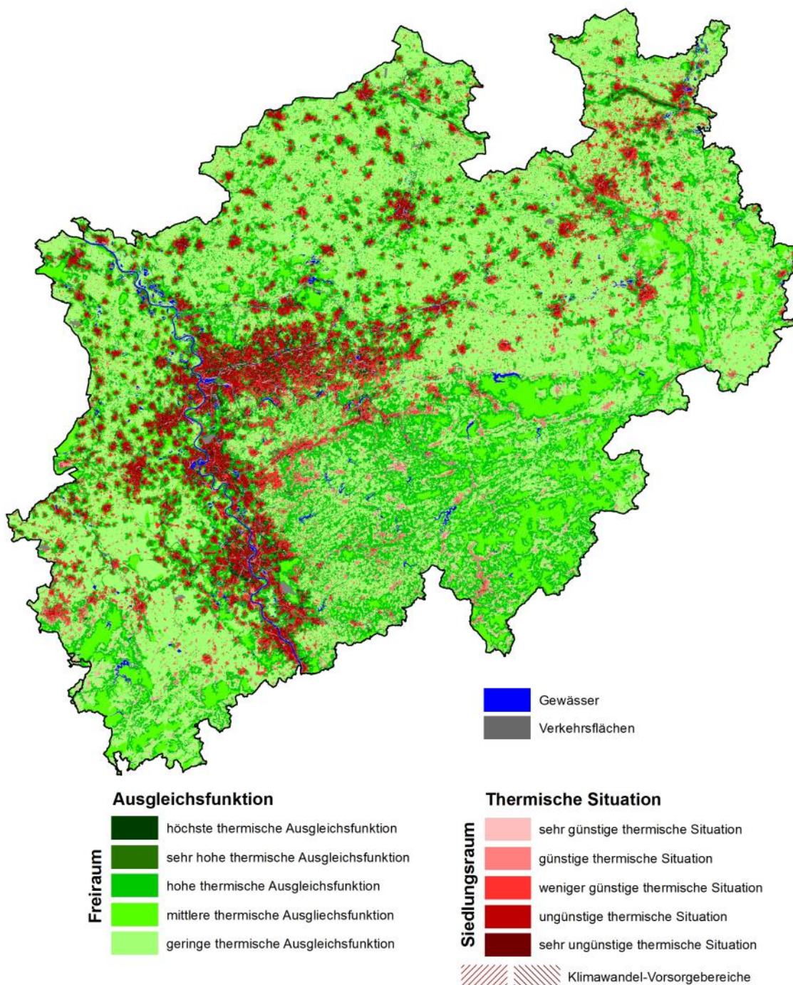
Abbildung 25: Klimaanalysekarte Gesamtbetrachtung
