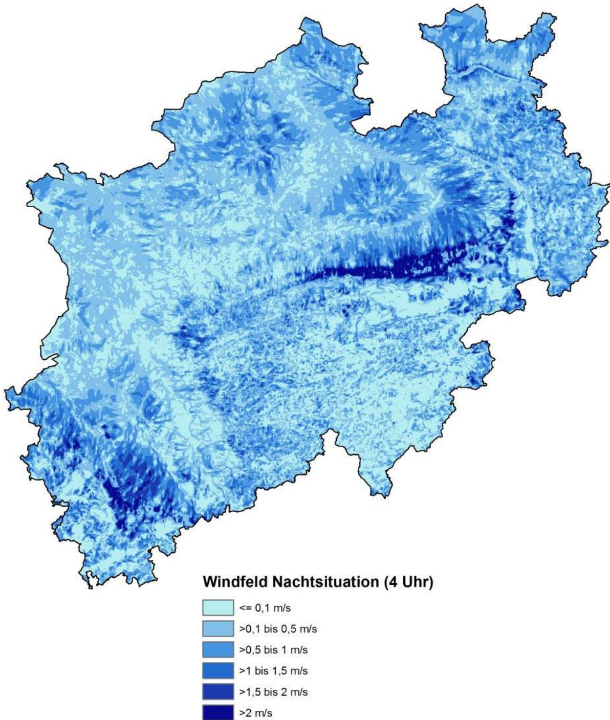
Abbildung 17: Nächtliches Windfeld
