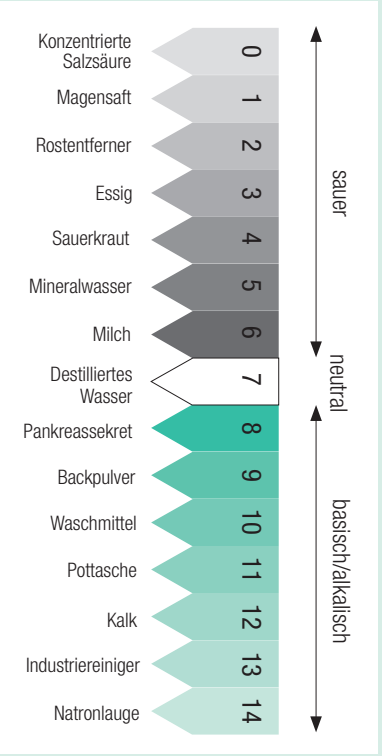
Von 0 bis 14: der pH-Wert am Beispiel verschiedener Stoffe.
