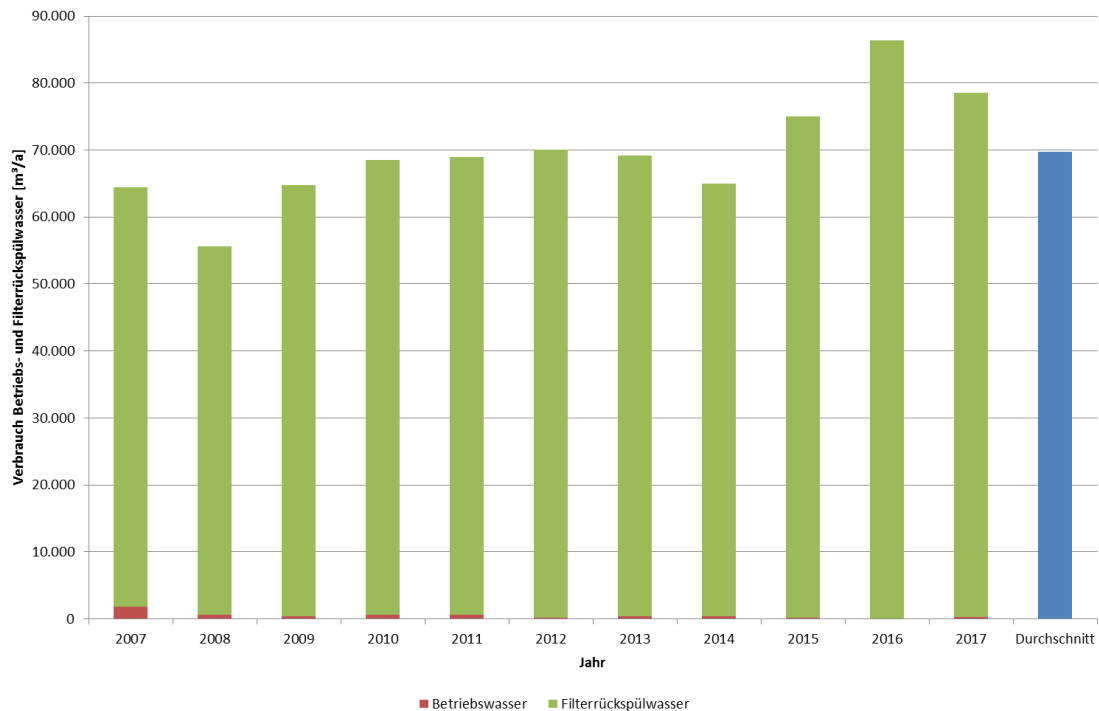
Abb. 7 Entwicklung des Trinkwassereigenbedarfs im Wasserwerk Vohen von 2007-2017
