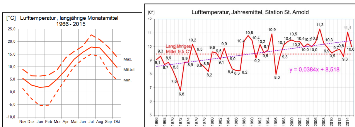
Abbildung 25: Jahresgang der monatlichen Lufttemperatur im langjährigen Mittel (links), mittlere jährliche Lufttemperatur von 1966 bis 2015 (rechts)
