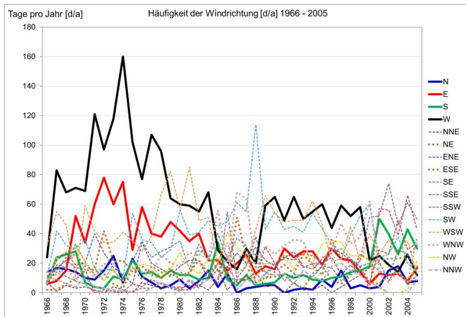
Abbildung 33: Entwicklung der Windrichtungen
