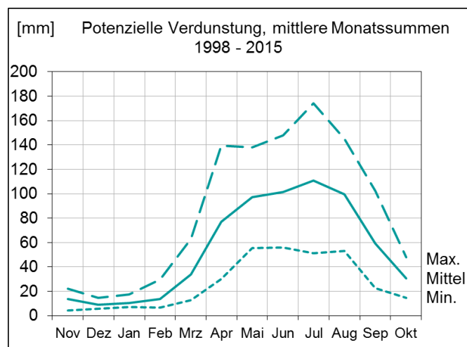
Abbildung 44: Jahresgang der potenziellen Verdunstung im Monatsmittel der Wasserversorgungsjahre von 1998 bis 2015
