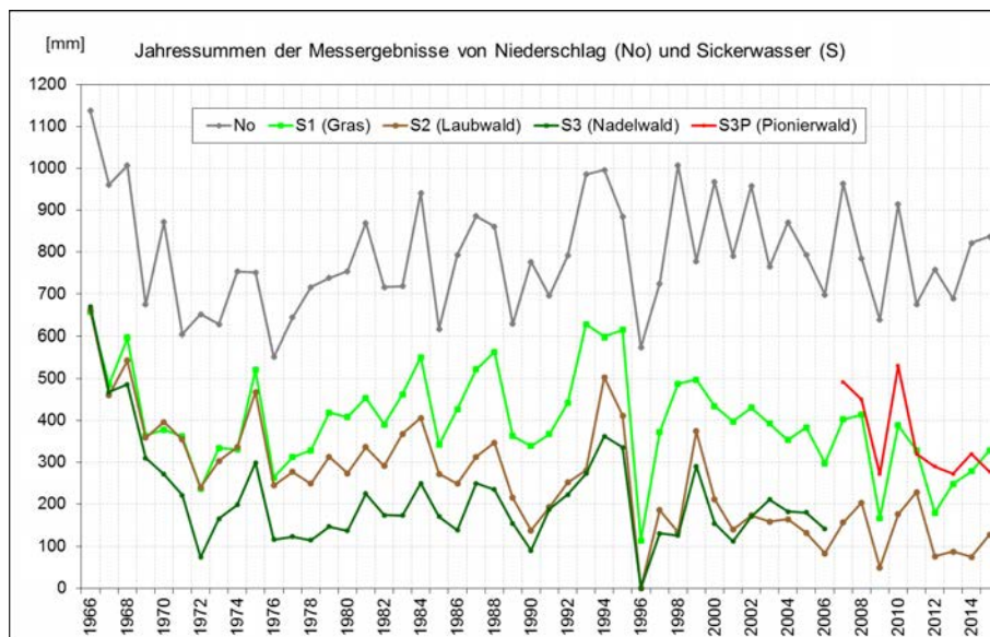
Abbildung 38: Messergebnisse von Niederschlag und Sickerwasser (NO: Niederschlag in Bodenhöhe gemessen)
