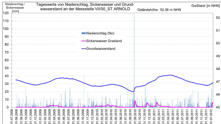
Abbildung 54: Tageswerte des Grundwasserstandes an der Messstelle VII/50_ST.ARNOLD, Nr. 110070501 sowie Tagessummen von Niederschlag und Sickerwasser am Grünland-Lysimeter
