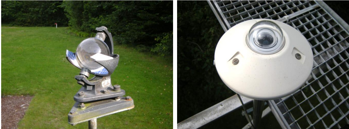
Abbildung 14: Sonnenschreiber (links), Globalstrahlungsmesser (rechts)
