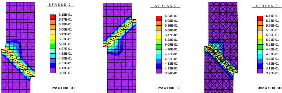
f. MES elem. g. EAS elem. h. CST and Mixed-CST elem.
