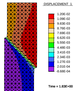
i. CST element.
