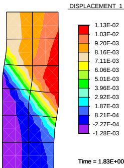
g. Q8 element.
