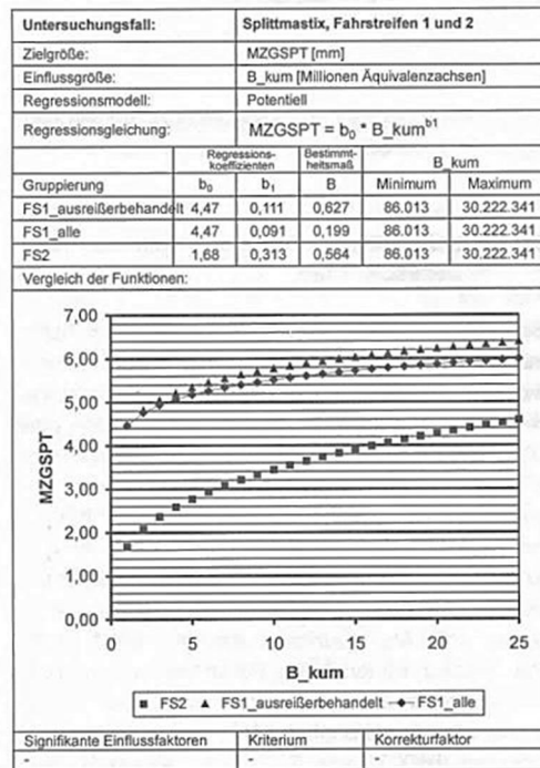
Abb. 32: Entwicklung der Spurrinnentiefe bei Splittmastix
