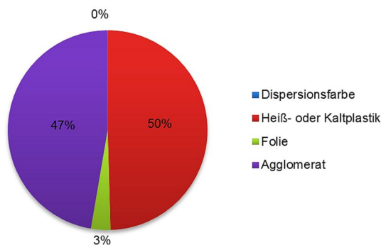
Abbildung 3-8: Prozentuale Verteilung der auf Autobahnen aufgetragenen Materialien für Straßenmarkierungen
