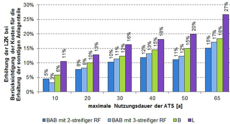
Abbildung 4-57: Relative Erhöhung der Lebenszykluskosten verschiedener Straßenkategorien bei Berücksichtigung der Kosten für die Erhaltung der sonstigen Anlagenteile
