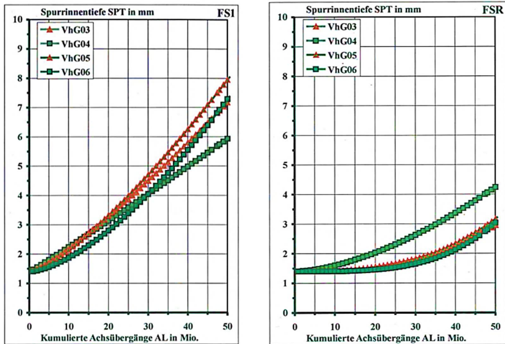
Abbildung 2-3: Verhaltensfunktionen für die Spurrinnentiefe verschiedener verhaltenshomogener Gruppen der Asphaltbauweise auf dem Hauptfahrstreifen (FS1) und den restlichen Fahrstreifen (FSR) [21]
