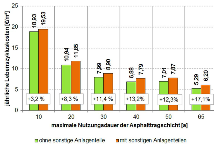
Abbildung 4-22: Auswirkungen der Kosten für die Erhaltung der sonstigen Anlagenteile auf die Lebenszykluskosten von Autobahnen mit 3-streifiger Richtungsfahrbahn
