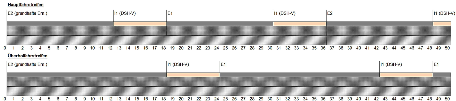
Abbildung 4-12: Erhaltungsstrategie für Autobahnen bei einer maximalen Nutzungsdauer der Asphalttragschicht von 40 Jahren auf dem Hauptfahrsstreifen
