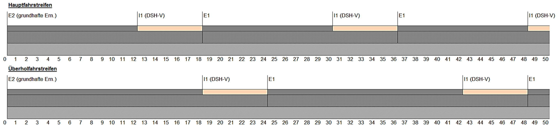
Abbildung 4-14: Erhaltungsstrategie für Autobahnen bei einer maximalen Nutzungsdauer der Asphalttragschicht von 65 Jahren auf dem Hauptfahrfahstreifen
