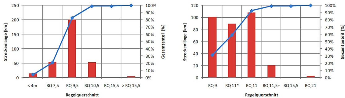
Abbildung 3-13: Streckenlänge und Summenlinie der vorhandenen Querschnitte (links) und der Querschnitte nach den RAL (rechts) [69]
