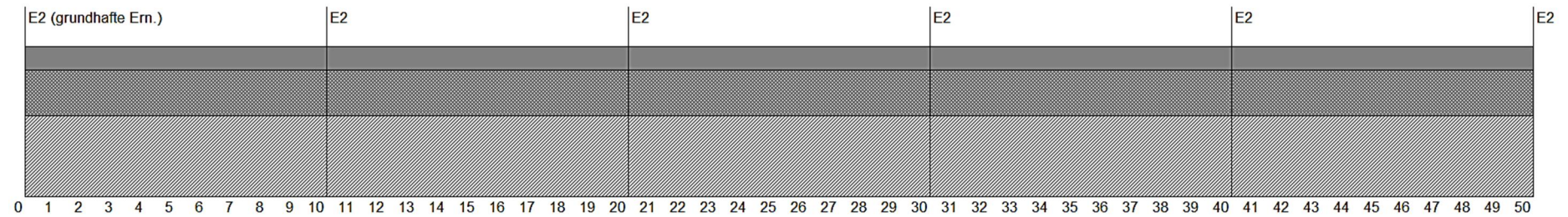
Abbildung 4-24: Erhaltungstrategie für Bundesstraßen bei einer maximalen Nutzungsdauer der Asphalttragschicht von 10 Jahren
