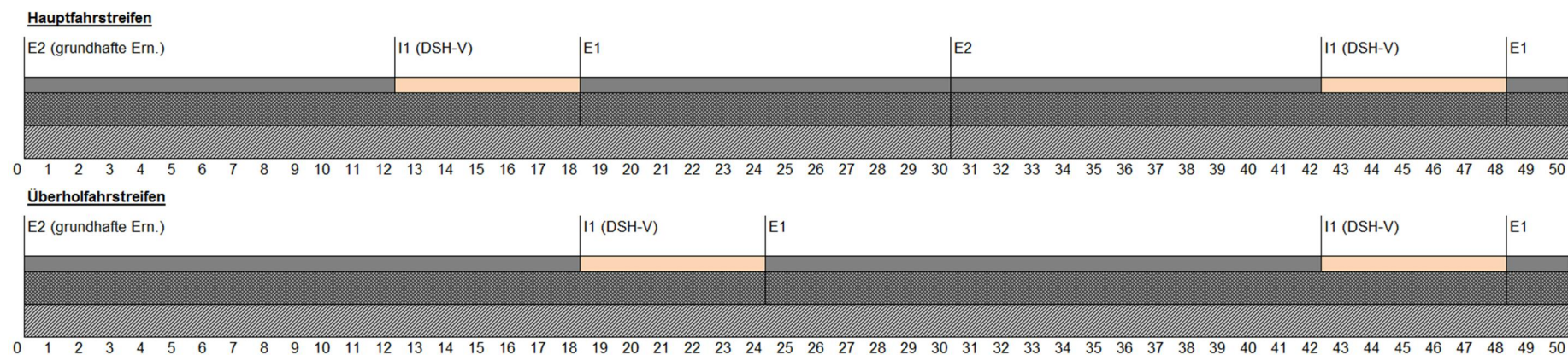
Abbildung 4-11: Erhaltungsstrategie für Autobahnen bei einer maximalen Nutzungsdauer der Asphalttragschicht von 30 Jahren auf dem Hauptfahrsstreifen
