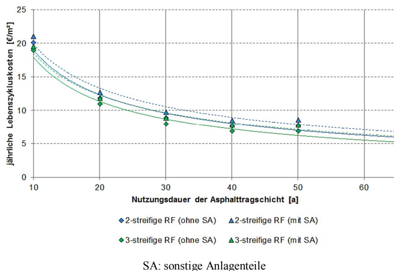
Abbildung 4-15: Jährliche Lebenszykluskosten von Autobahnen in Abhängigkeit von der maximalen Nutzungsdauer der Asphalttragschicht
