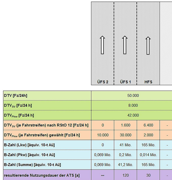
Abbildung 3-36: Vorüberlegung zur Verteilung des DTV auf die Fahrstreifen einer Autobahn mit 3-streifiger Richtungsfahrbahn
