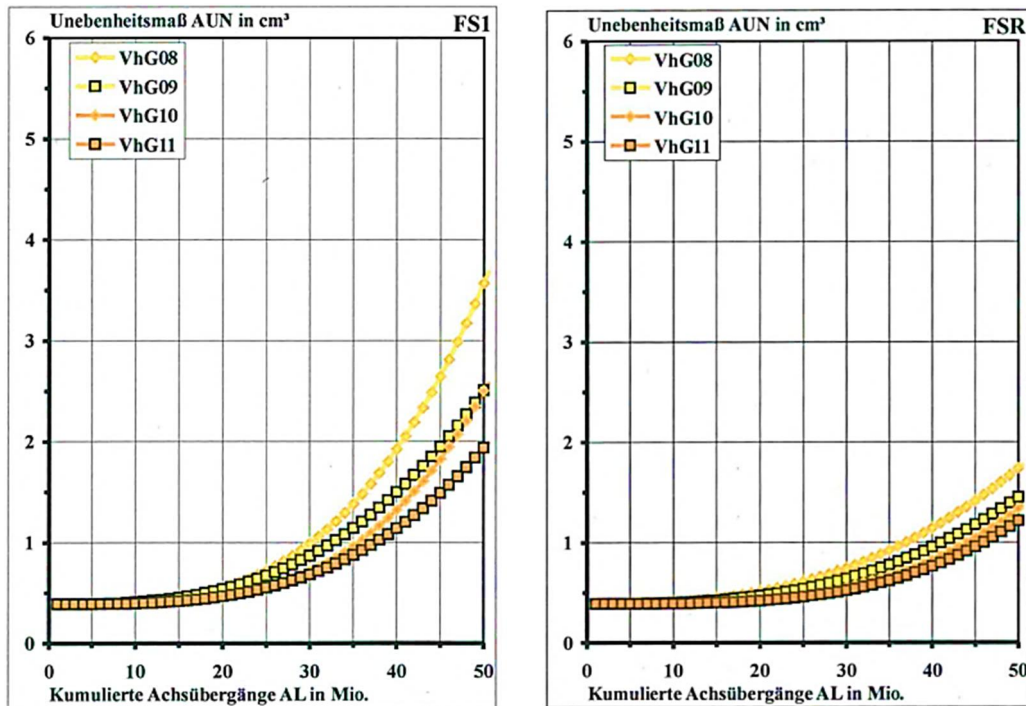
Abbildung 2-4: Verhaltensfunktionen für das Unebenheitsmaß AUN verschiedener verhaltenshomogener Gruppen der Betonbauweise auf dem Hauptfahrstreifen (FS1) und den restlichen Fahrstreifen (FSR) [21]
