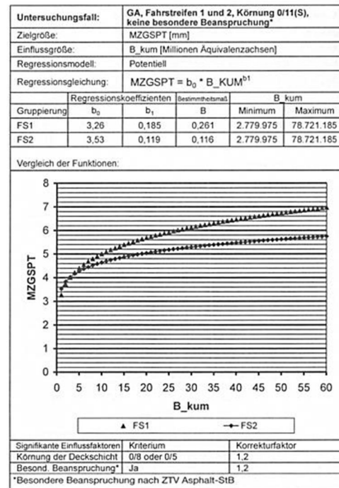
Abb. 29: Entwicklung der Spurrinnentiefe bei Gussasphalt
