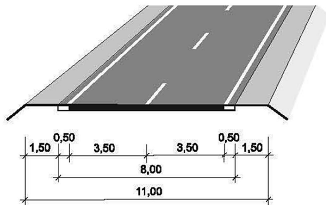
Abbildung 3-14: Gewählter Regelquerschnitt für Bundesstraßen gemäß den RAL
