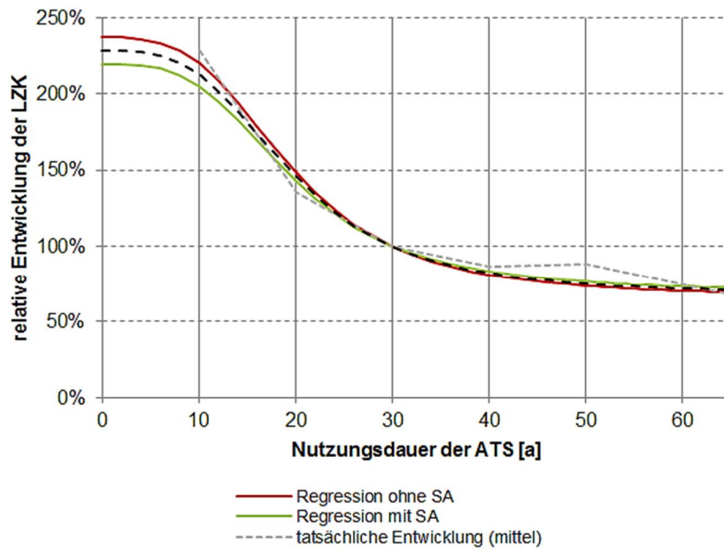
Abbildung 4-17: Relative Entwicklung der Lebenszykluskosten von Autobahnen mit 3-streifiger Richtungsfahrbahn in Abhängigkeit von der Nutzungsdauer der Asphalttragschicht
