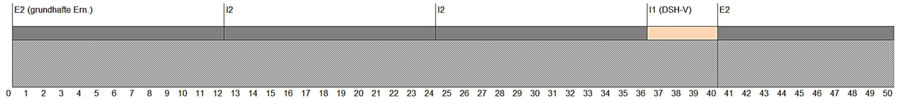
Abbildung 4-42: Erhaltungstrategie für Landesstraßen bei einer maximalen Nutzungsdauer der Asphalttragschicht von 40 Jahren
