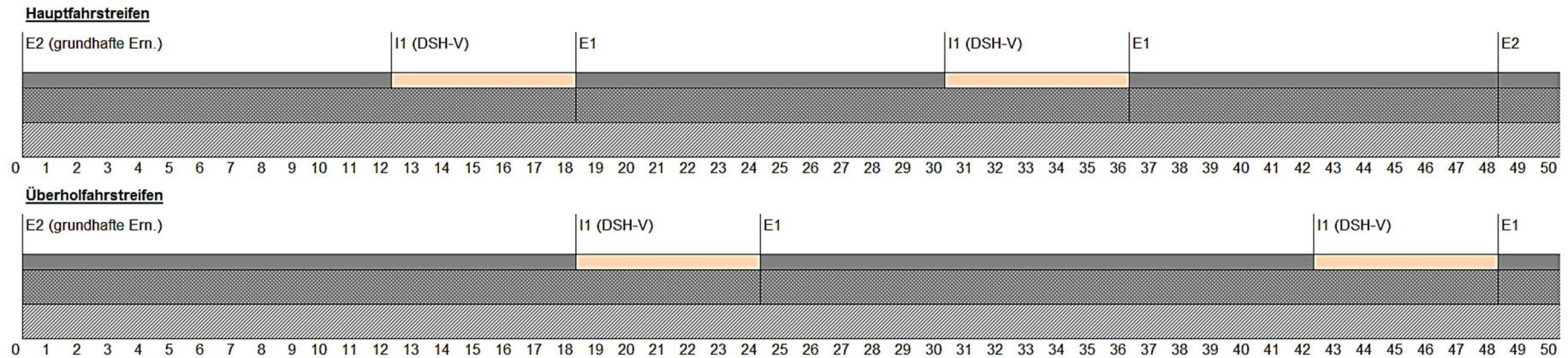
Abbildung 4-13: Erhaltungsstrategie für Autobahnen bei einer maximalen Nutzungsdauer der Asphalttragschicht von 50 Jahren auf dem Hauptfahrfahstreifen
