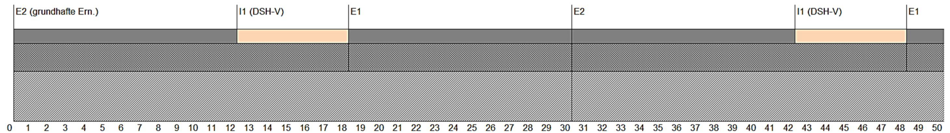
Abbildung 4-26: Erhaltungstrategie für Bundesstraßen bei einer maximalen Nutzungsdauer der Asphalttragschicht von 30 Jahren
