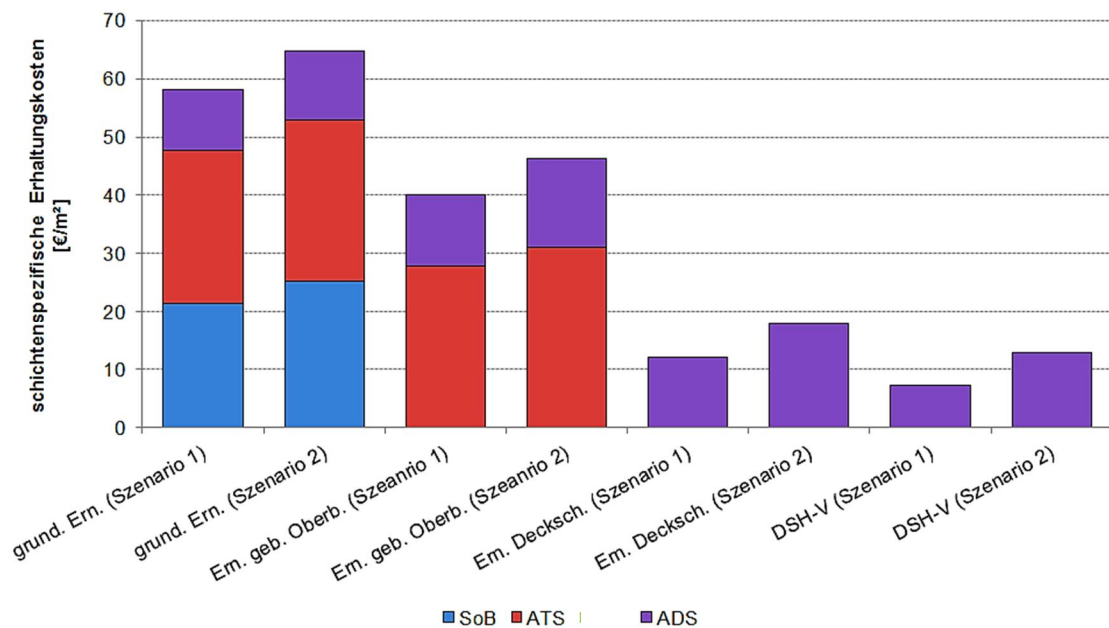
Abbildung 3-33: Schichtenspezifische Kosten [€/m²] für die Erhaltungsmaßnahmen an Landesstraßen
