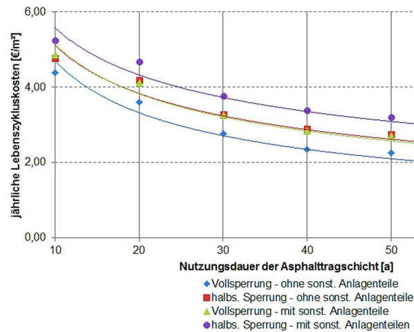
Abbildung 4-45: Entwicklung der Lebenszykluskosten von Landesstraßen in Abhängigkeit von der Nutzungsdauer der Asphalttragschicht
