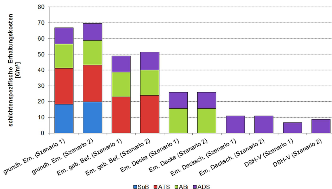
Abbildung 3-32: Schichtenspezifische Kosten [€/m²] für Erhaltungsmaßnahmen an Bundesstraßen
