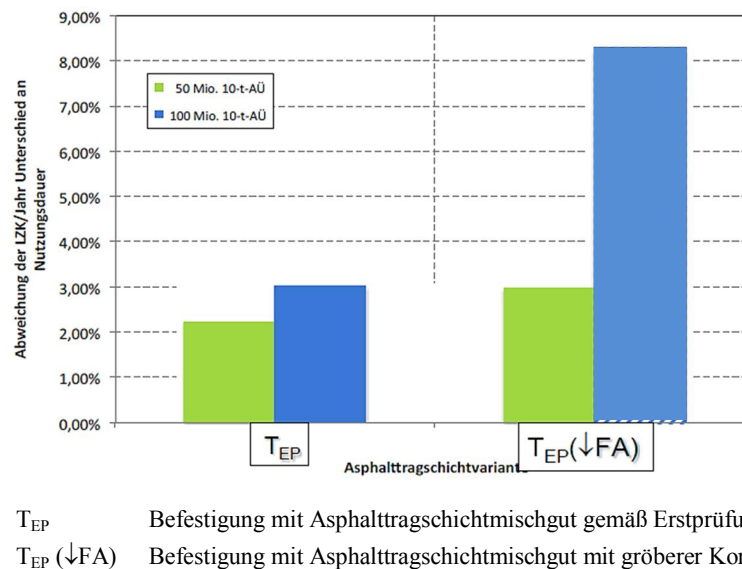
Abbildung 5-7: Einfluss einer von der Dimensionierung abweichenden Nutzungsdauer am Bohrkern auf die jährlichen Lebenszykluskosten [5]
