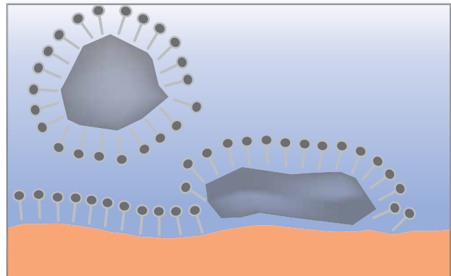
Abb. 3.2. Tenside lagern sich mit ihrem hydrophoben Ende an die Feststoffe an und lösen lockere Partikel ab.
