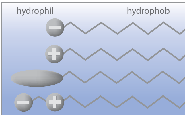
Abb. 3.1. Je nach Ladung ist das Tensid anionisch, kationisch, nichtionisch oder amphoter.
