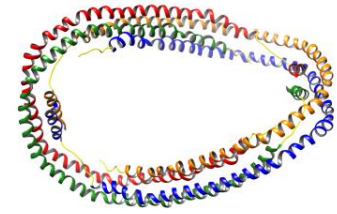
Fig. 1: Apolipoprotein A1
