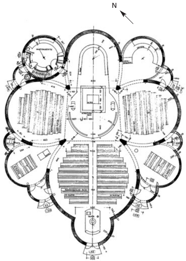
4 Grundriss der Kirche.
