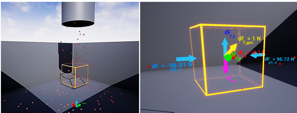
Abbildung 4: Differentielles Volumenelement (gelb) zur Herleitung von Erhaltungsgleichungen in einer Strömung (links), mit zugeschalteten Kräften und Zahlenwerten (rechts)
