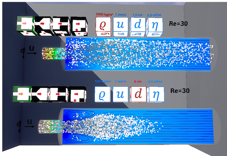
Abbildung 2: Scheinbar unterschiedlich schnelle Partikel bei dennoch gleichem Strömungsverlauf
