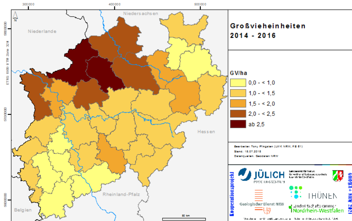
Abbildung 2-6: Großvieheinheitenbesatz
