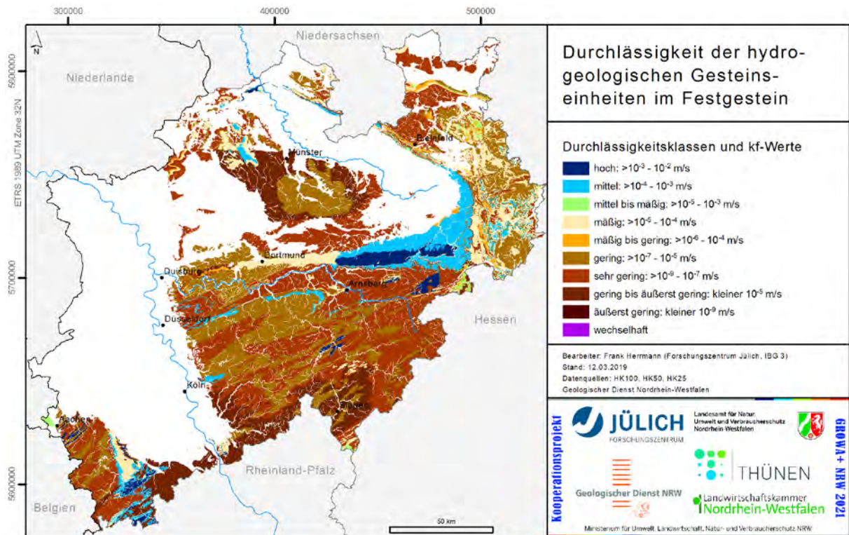
Abb. 20: Durchlässigkeit der hydrogeologischen Gesteinseinheiten im Festgestein
