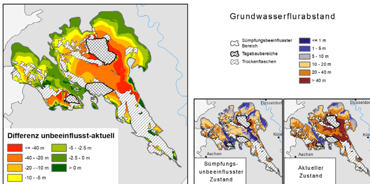
Abb. 9-1: Änderungen im Flurabstand des Grundwassers
