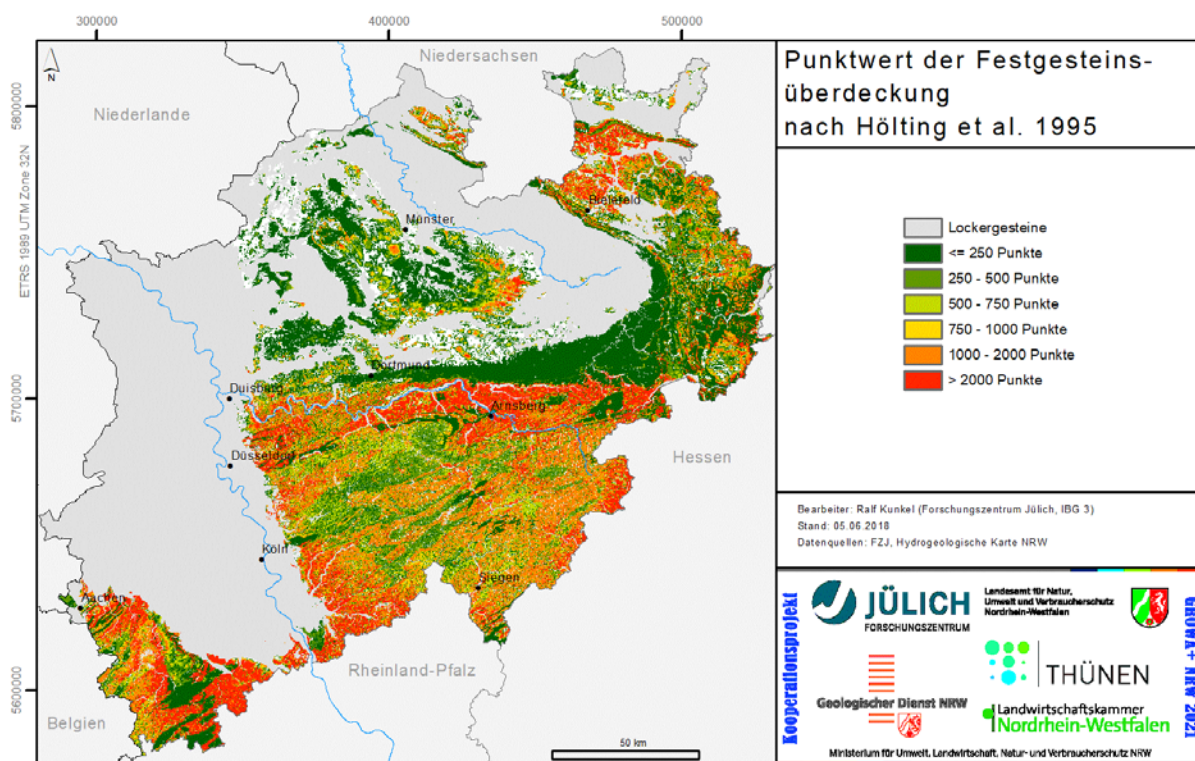
Abb. 6-3: Punktwert der Festgesteinsüberdeckung nach Hölting et al. (1995)
