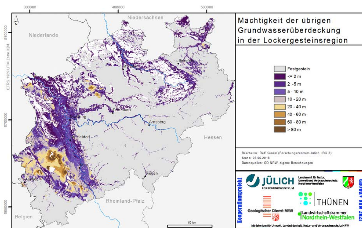
Abb. 5-11: Mächtigkeit der „übrigen“ Grundwasserüberdeckung in der Lockergesteinsregion
