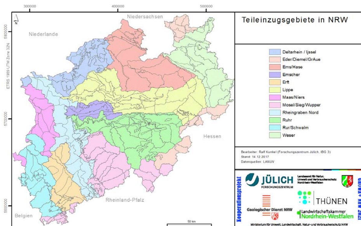
Abb. 10-3: Teileinzugsgebiete NRW
