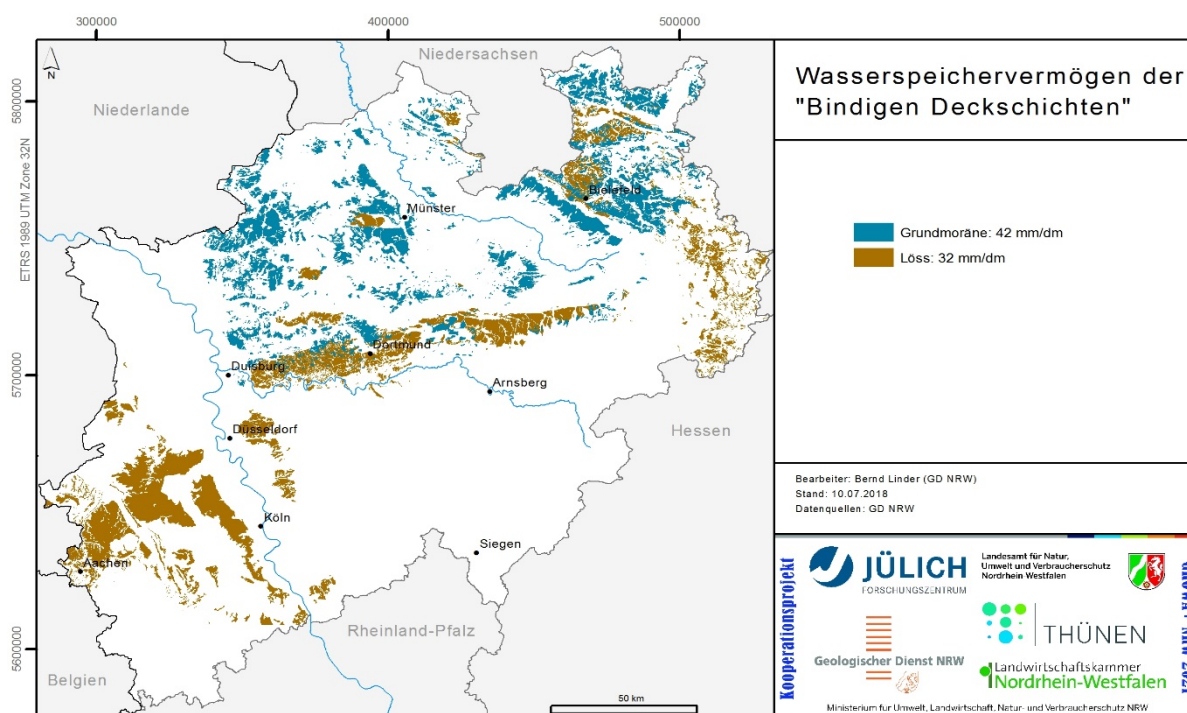
Abb. 5-11: Wasserspeichervermögen der Bindigen Deckschichten
