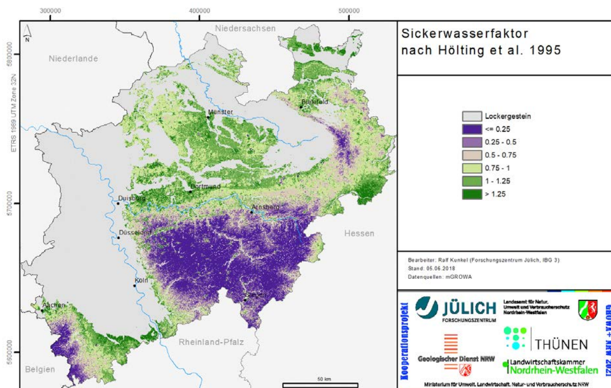
Abb. 5-16: Sickerwasserfaktor nach Hölting
