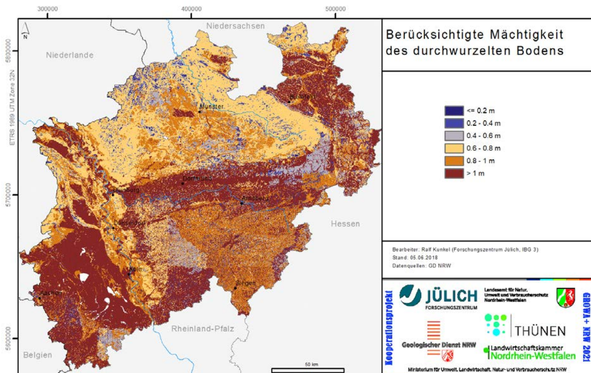
Abb. 5-1: Berücksichtigte Mächtigkeit des durchwurzelten Bodens
