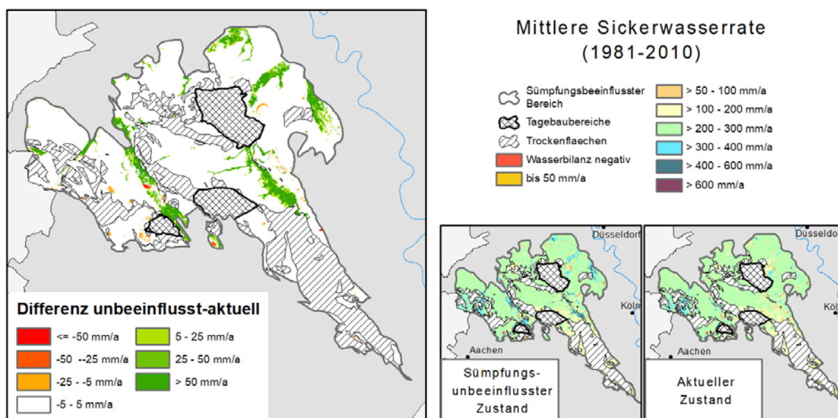
Abb. 9-2: Änderungen in der Sickerwasserrate
