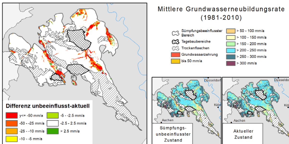
Abb. 9-3: Änderungen in der Grundwasserneubildungsrate
