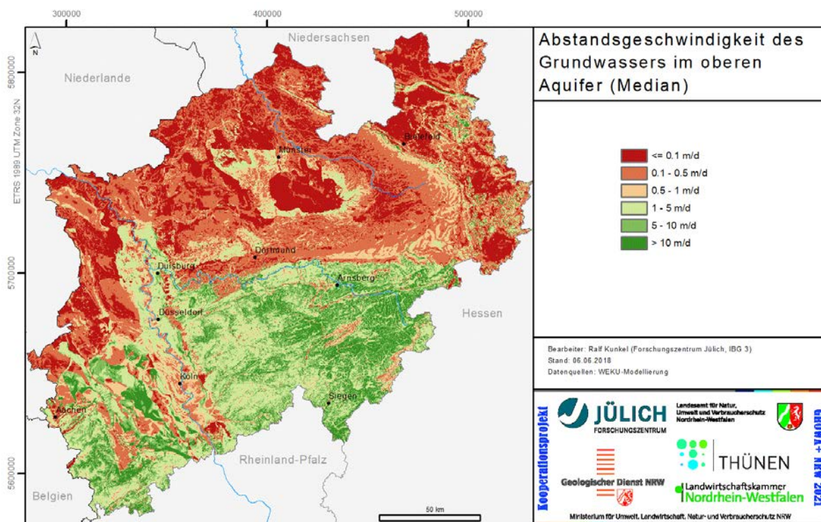
Abb. 7-1: Abstandsgeschwindigkeit des Grundwassers im oberen Aquifer
