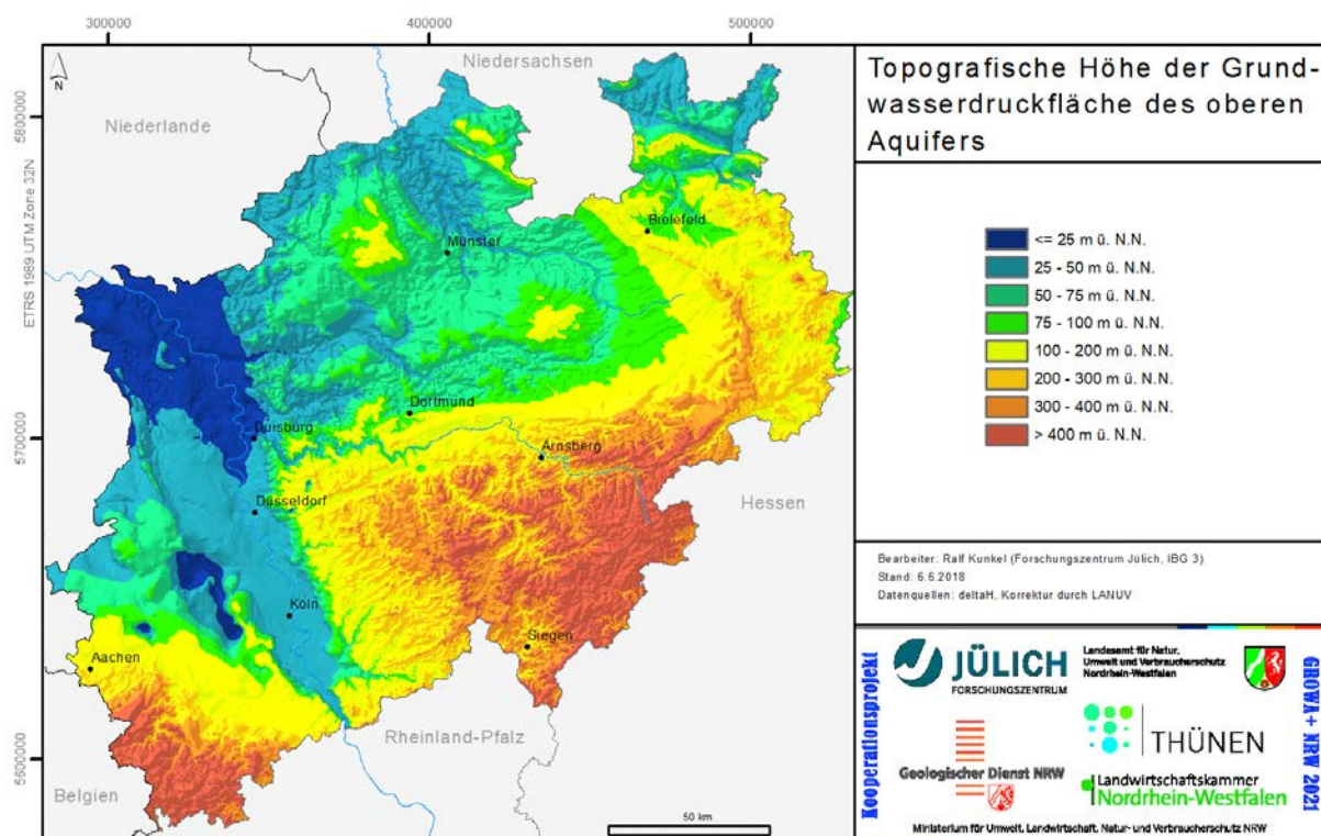
Abb. 5-5: Digitales Modell der Grundwasseroberfläche NRW (König & König, 2017)
