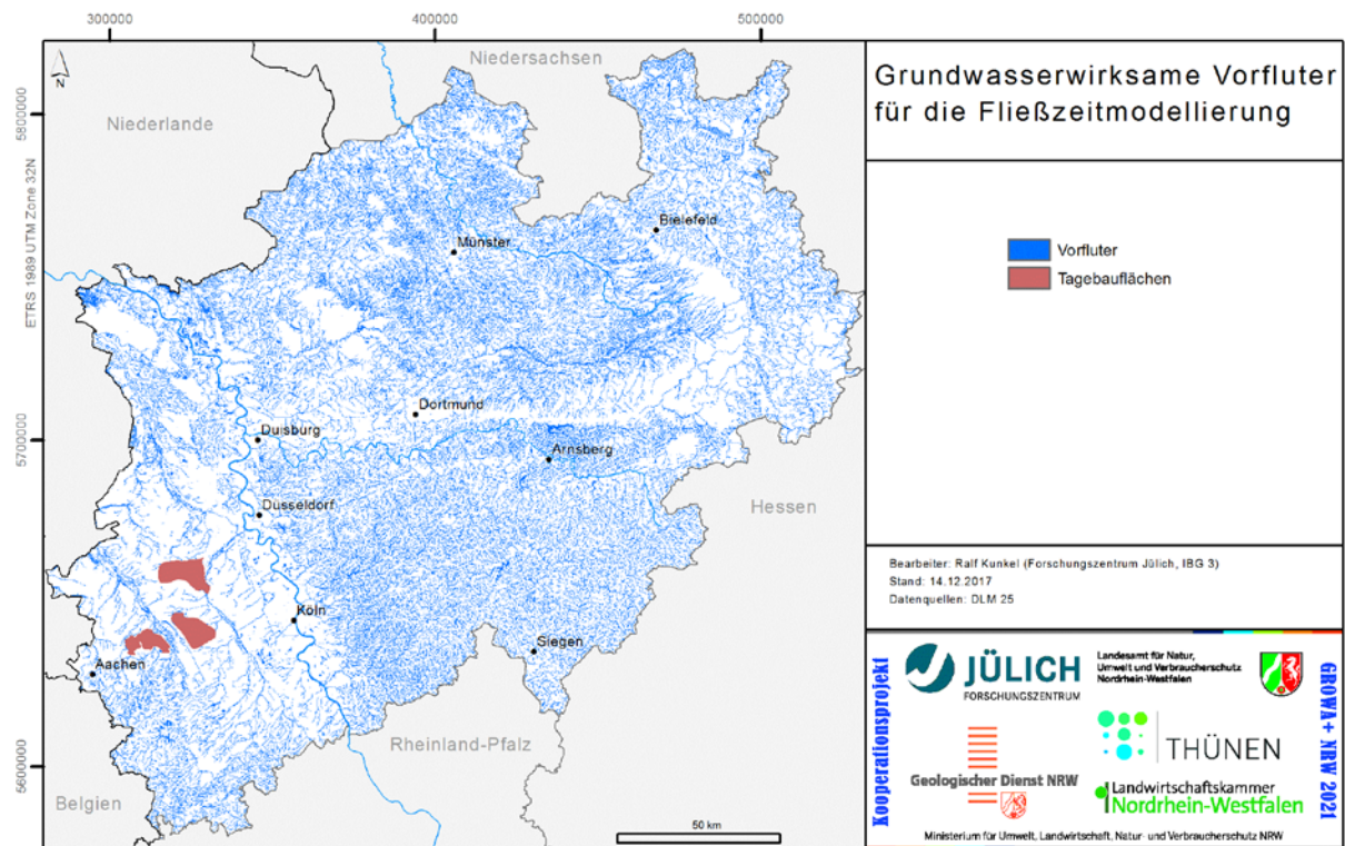
Abb. 5-9: Grundwasserwirksame Vorfluter
