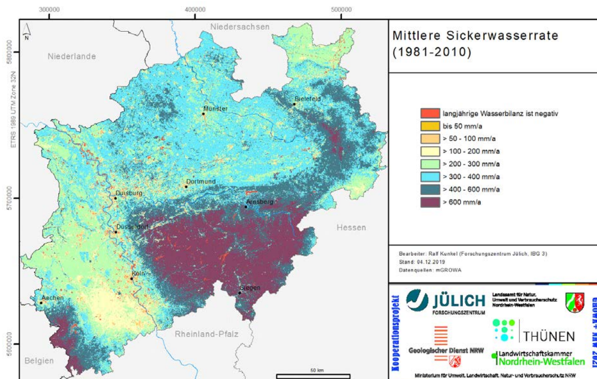
Abb. 5-21: Sickerwasserrate 1981-2010 nach mGROWA
