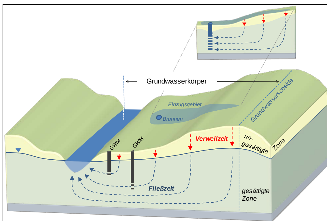
Abb. 1-2: Räumlicher Bezug für die Verweil- und Fließzeitermittlung auf GWK-Ebene sowie bis Vorflutereintritt (Hansen et al., 2018)
