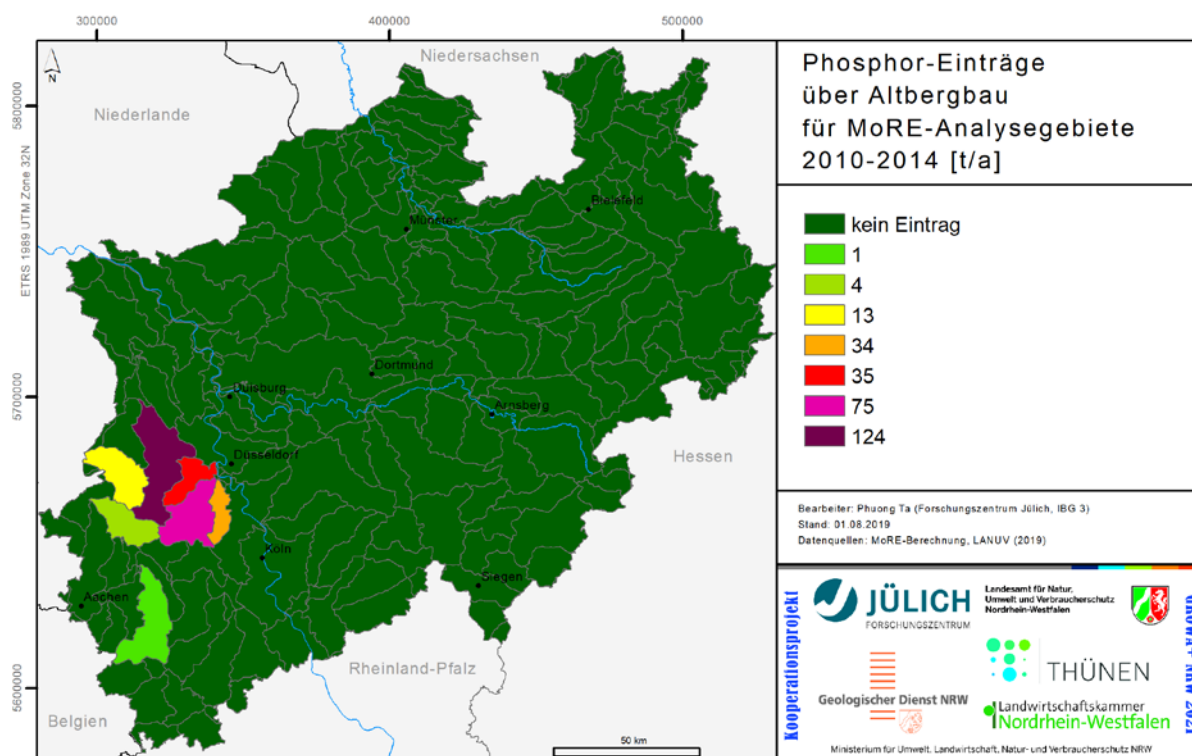
Abb. 4-12: Mittlere Phosphor-Einträge aus (Alt-)Bergbau
