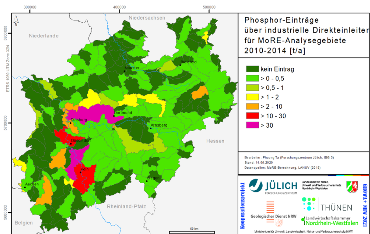
Abb. 4-8: Mittlere Phosphor-Einträge aus industriellen Direkteinleitungen
