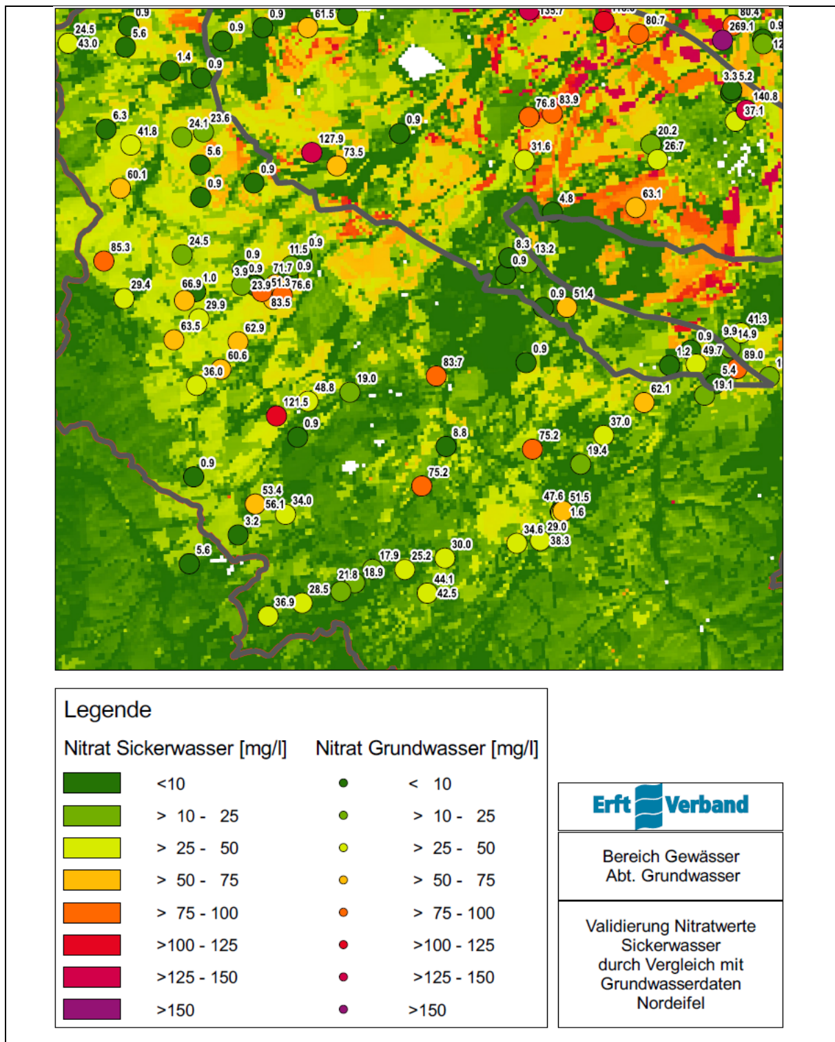
Abb. 3-14: Vergleich der modellierten mittleren langjährigen Nitratkonzentration im Sickerwasser (Flächenfarben) mit gemessenen Nitratkonzentrationen im Grundwasser (Punktfarben) für die Nordeifel: Mechernicher Triasbucht (Nordwesten) und Sötenicher Kalkmulde (Süden)
