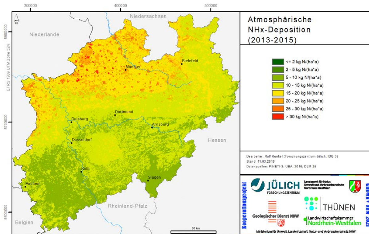
Abb. 2-3: Mittlere mehrjährige atmosphärische NH x -Deposition
