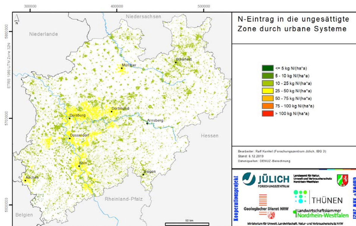
Abb. 2-7: N-Austräge aus urbanen Systemen
