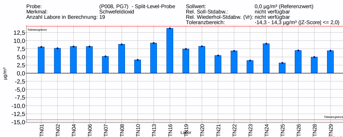
Abbildung 25: Schwefeldioxid-Konzentration ca. 30 µg/m³ - Störkomponente NO ca. 500 nmol/mol
