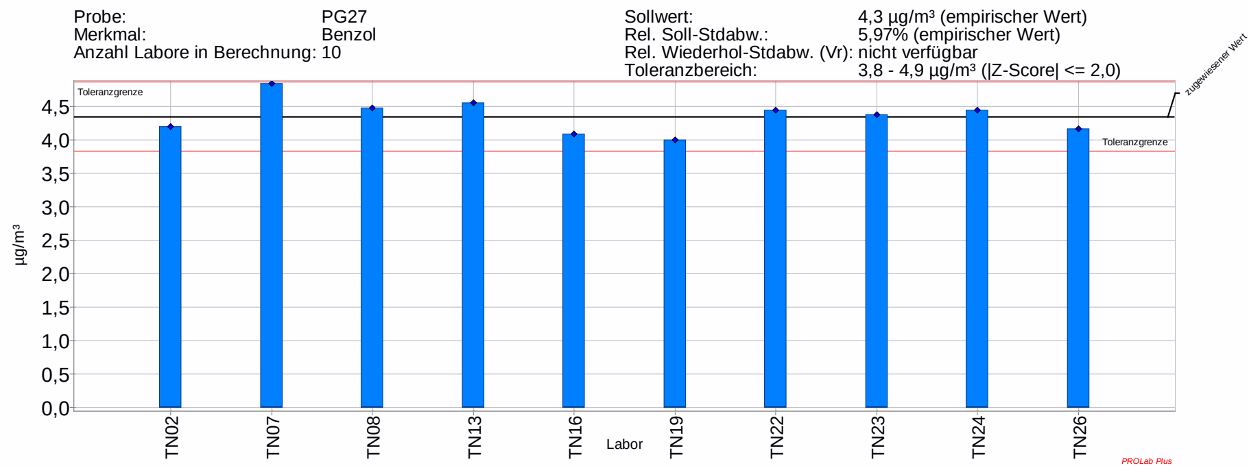
Abbildung 15: Prüfgasangebot 27 - Komponente Benzol
