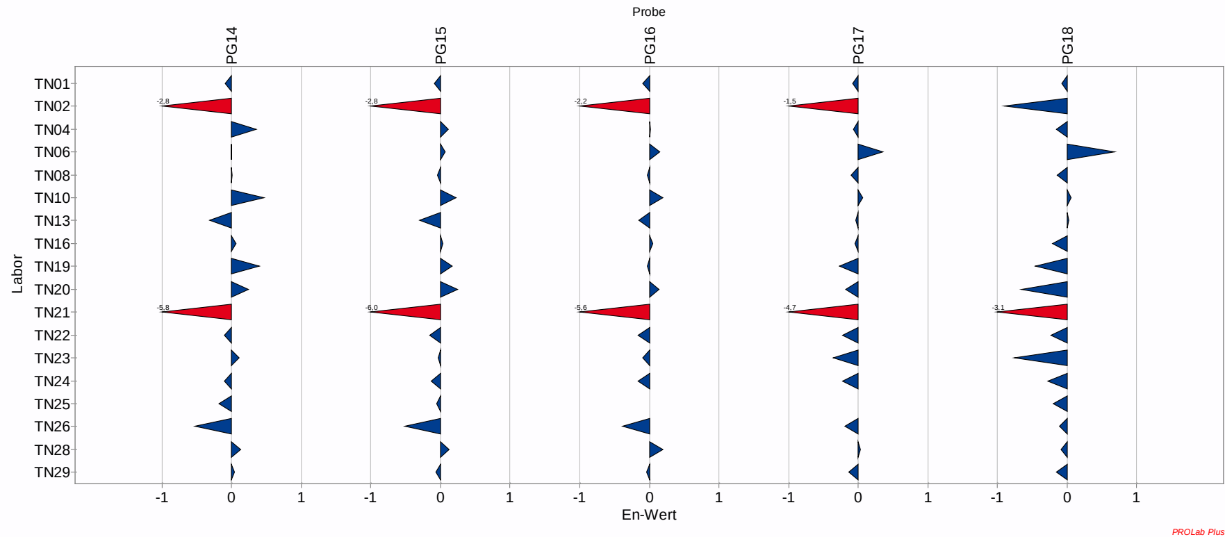
Abbildung 18 En-Zahlen Schwefeldioxid
