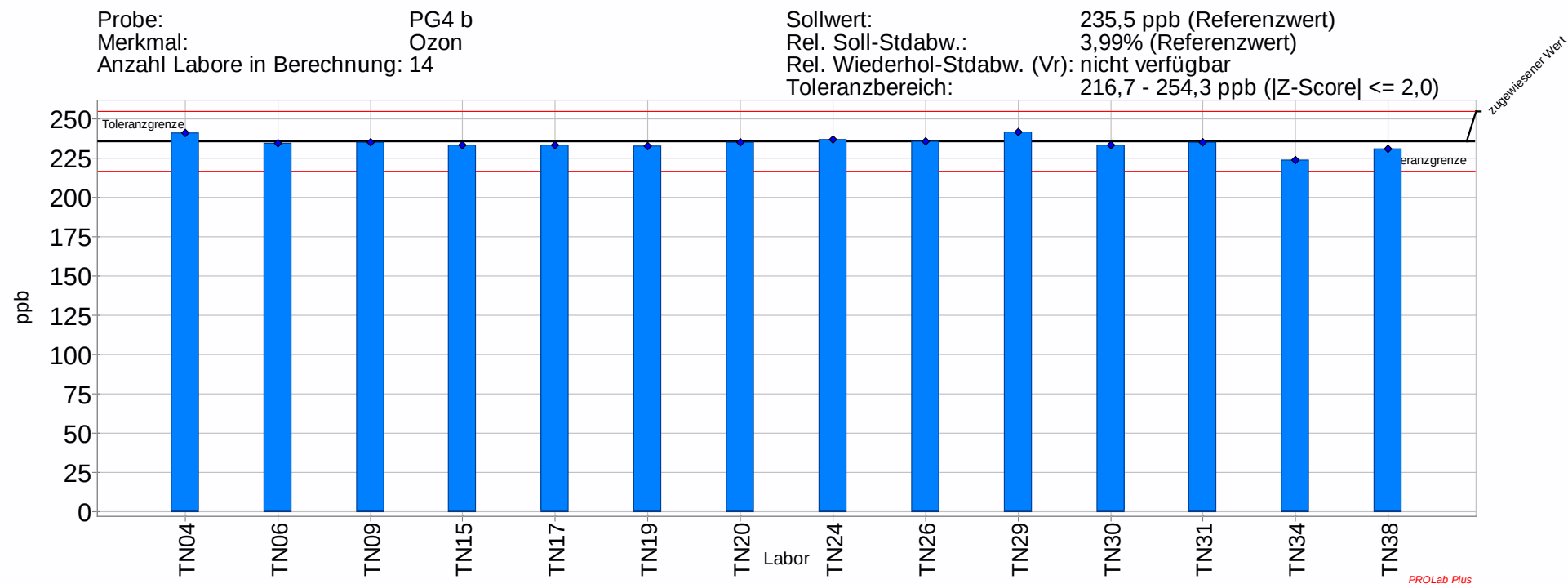
Abbildung 25: Prüfgasangebot 4 b Komponente Ozon
