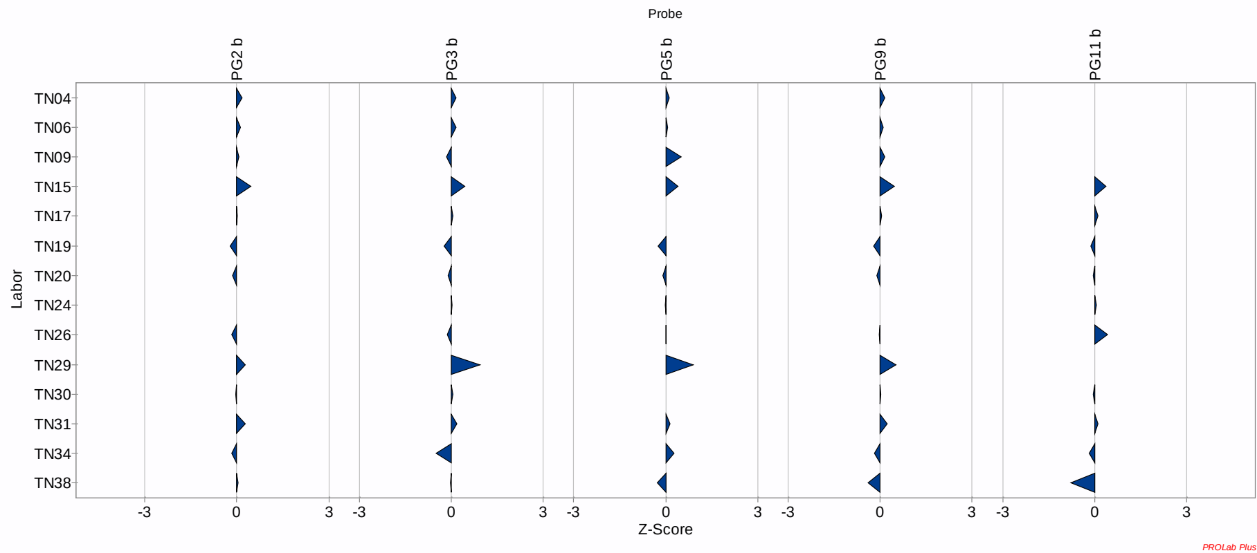
Abbildung 36: z'-score Übersicht Stickstoffmonoxid Gruppe II
