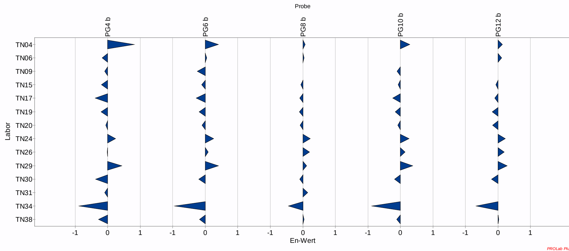
Abbildung 41: E_n -Zahlen Ozon Gruppe II
