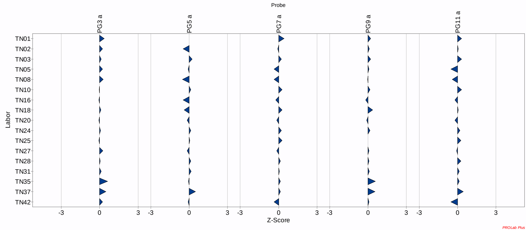
Abbildung 6: z'score Übersicht Gruppe I Stickstoffdioxid
