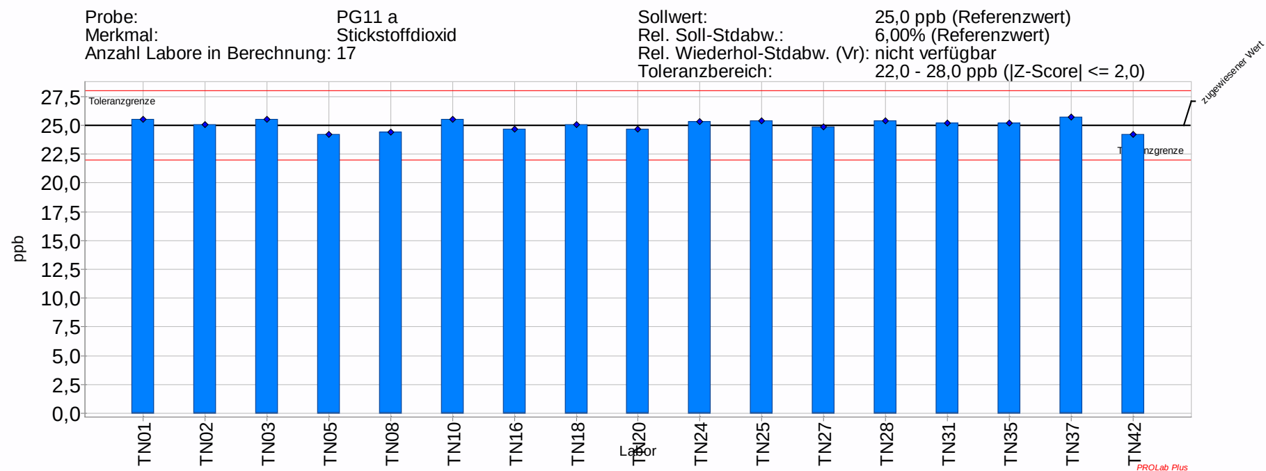
Abbildung 5: Prüfgasangebot 11 a Komponente Stickstoffdioxid
