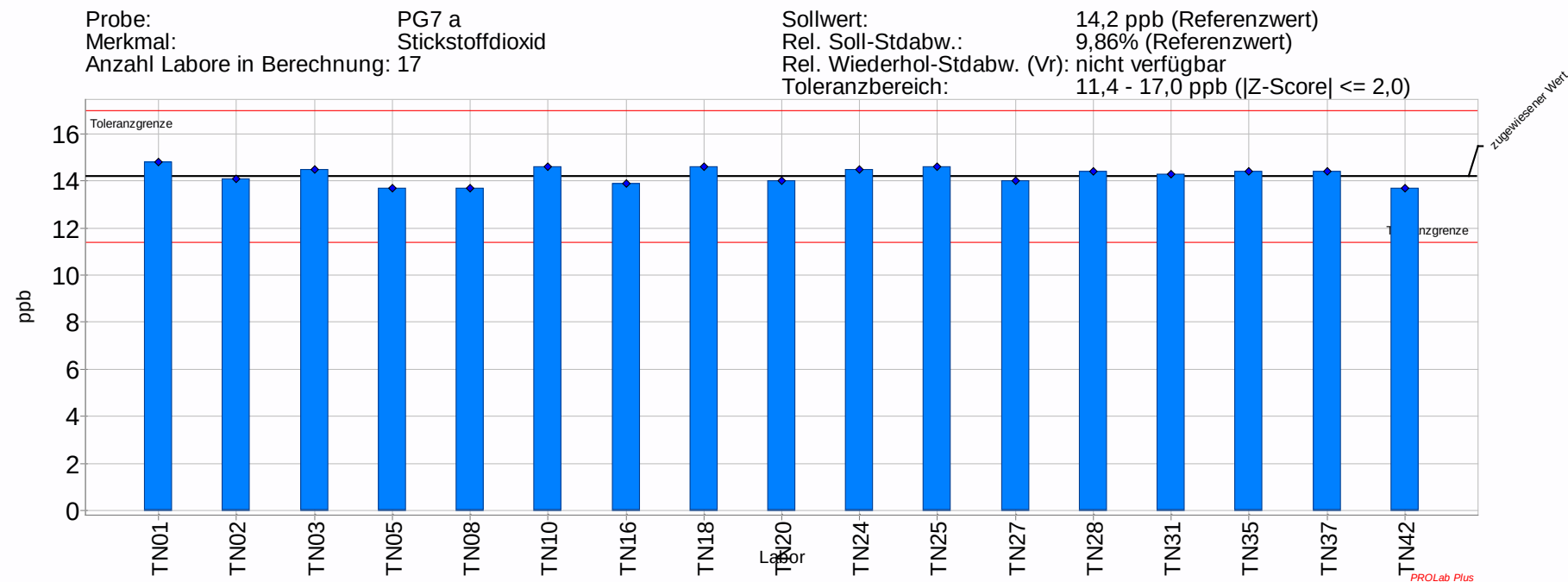
Abbildung 3: Prüfgasangebot 7 a Komponente Stickstoffdioxid
