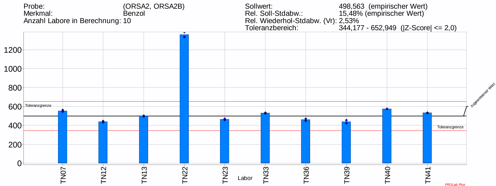
Abbildung 44: Robuste Auswertung Benzol – Doppelbestimmung Probe ORSA 2
