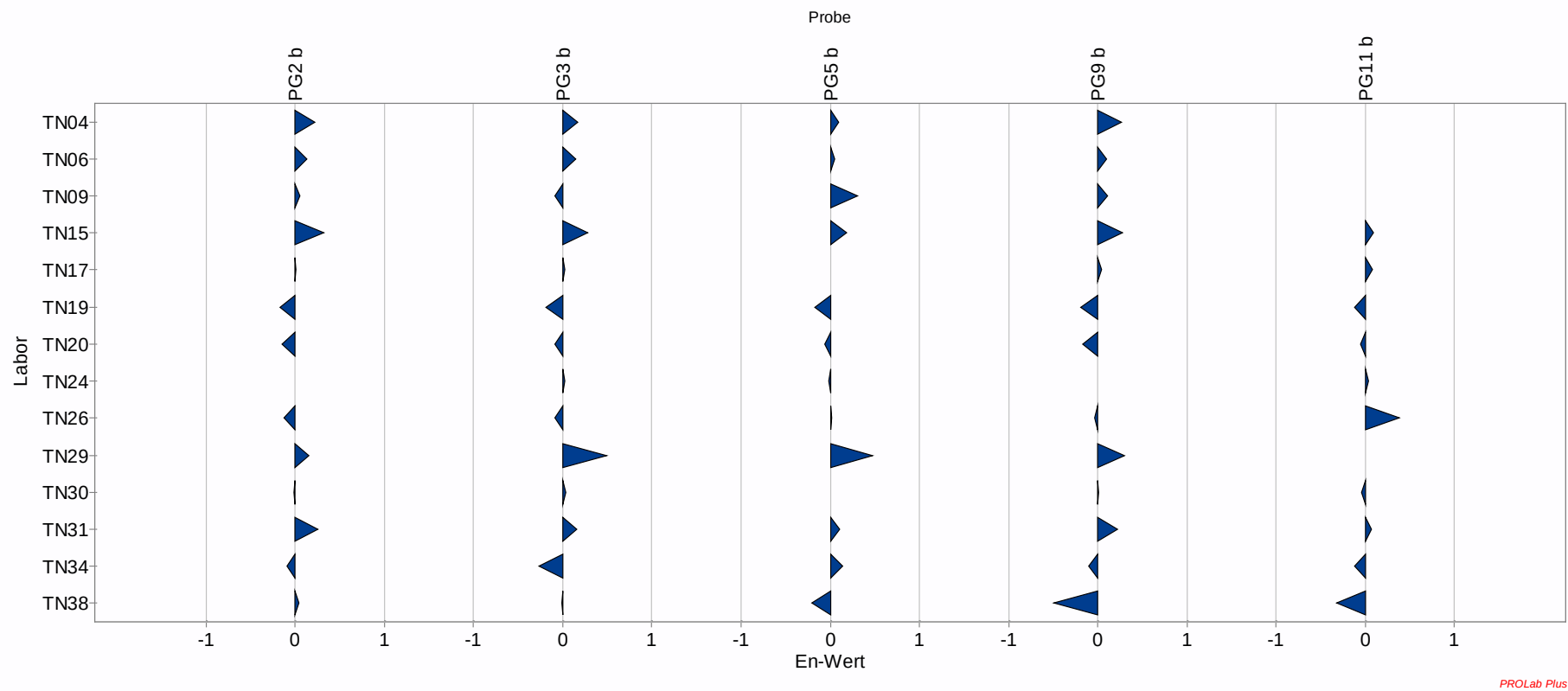
Abbildung 42: E n -Zahlen Stickstoffmonoxid Gruppe II
