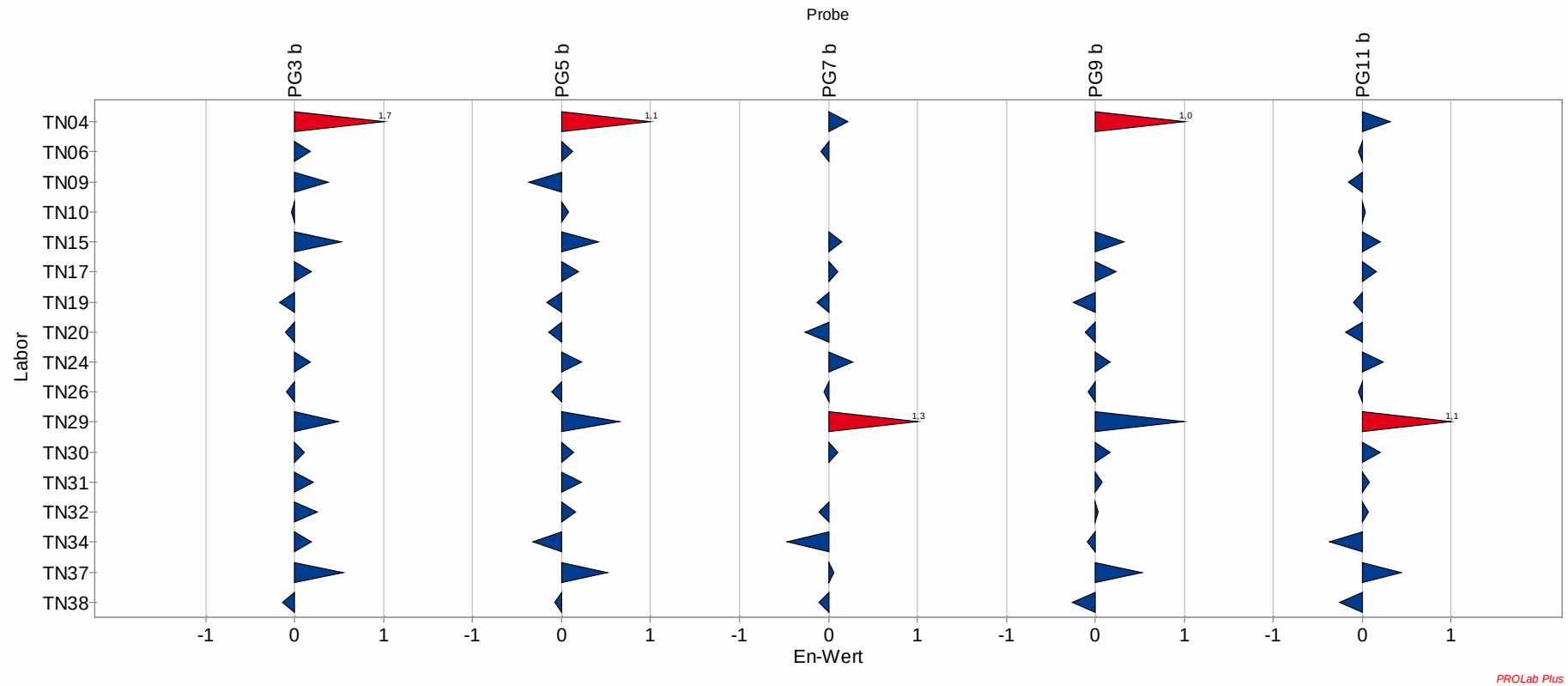
Abbildung 40: En-Zahlen Stickstoffdioxid Gruppe II
