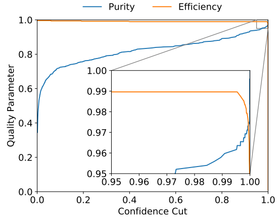
(d) LSTM
