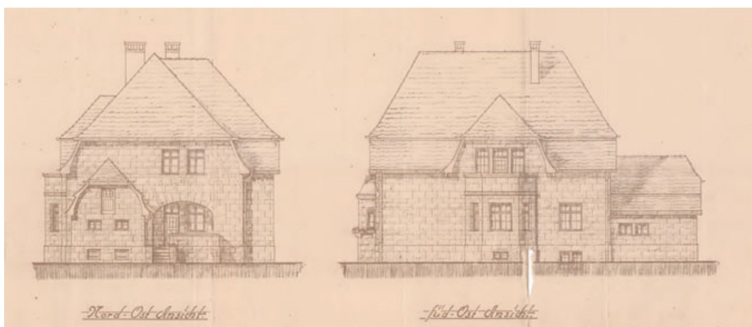
2 Die Ansichtszeichnungen aus dem Bauantrag zeigen die durchdachte Baustruktur und die hohe Bedeutung der Materialität für das Bauprojekt.
