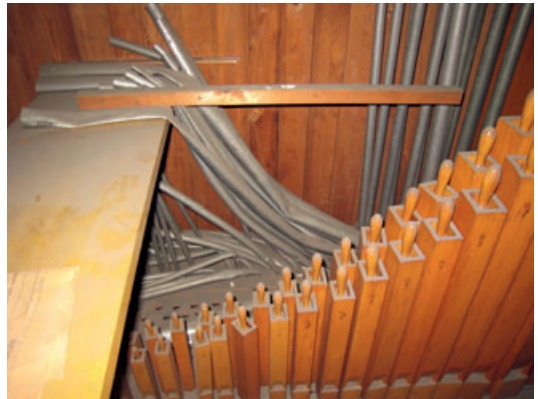
9 Geschädigtes Pfeifenwerk des Echowerks. Foto 2018.
